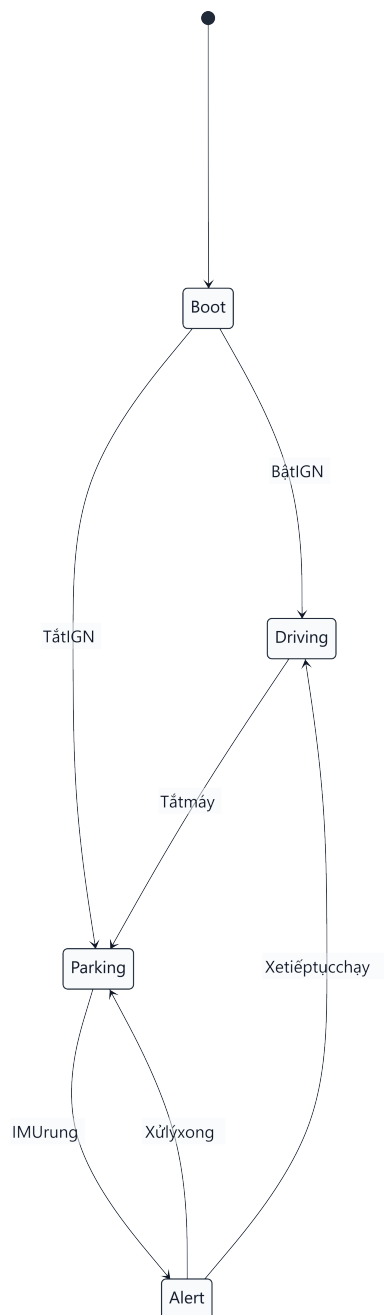
Hình 3.11: Sơ đồ máy trạng thái của thiết bị theo dõi
