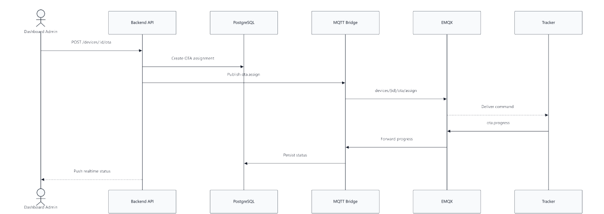
Hình 3.14a: Luồng điều phối OTA giữa Backend, EMQX, thiết bị và MQTT Bridge
