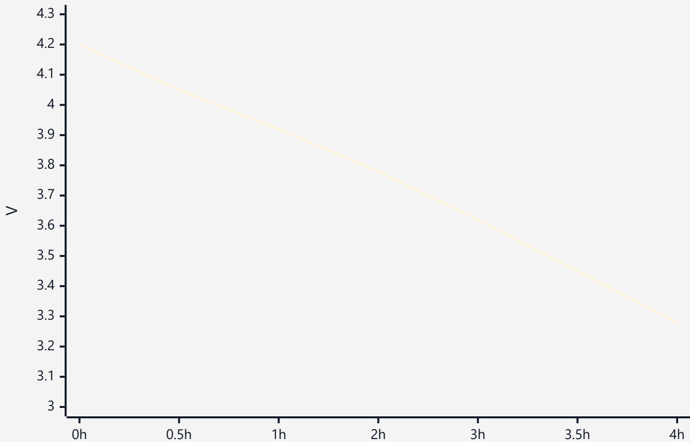
Điện áp pin dự phòng theo thời gian
