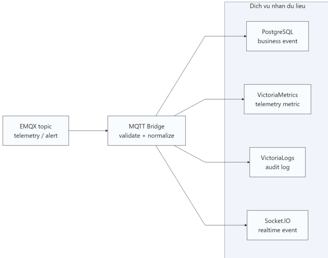
Hình 4.20: Luồng xử lý dữ liệu của MQTT Bridge
