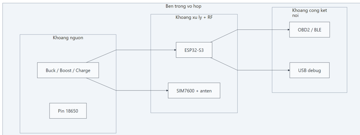
Hình 4.11: Sơ đồ bố cục bên trong vỏ hộp bảo vệ
