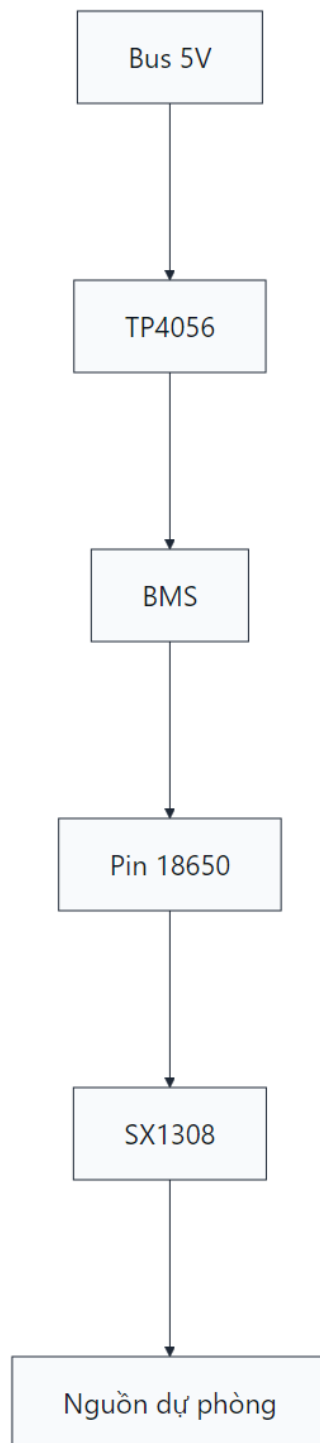
Hình 4.10: Kiến trúc sạc pin TP4056 và đường cấp nguồn dự phòng
