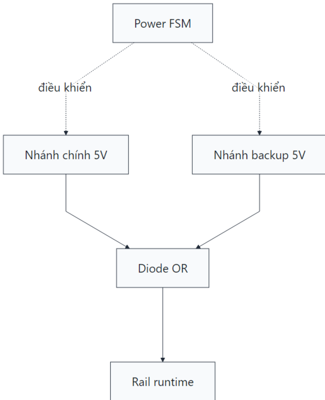
Hình 4.9: Sơ đồ power path runtime giữa nhánh chính và nhánh backup
