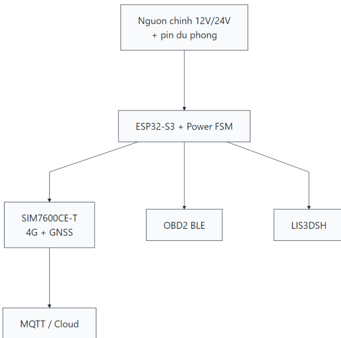
Hình 4.1: Sơ đồ khối tổng thể hệ thống tracker IoT
