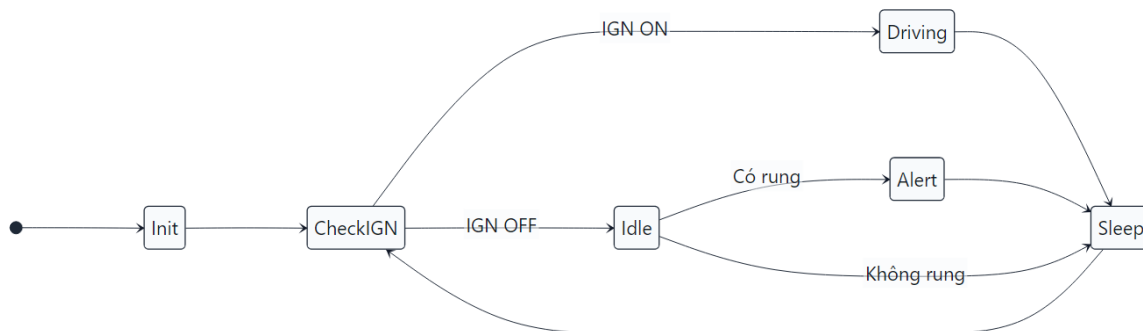
Hình 3.7: Lưu đồ thuật toán luồng hoạt động chính của firmware
