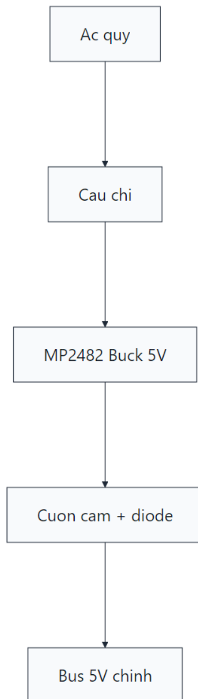
Hình 4.7: Kiến trúc nhánh buck 5V chính dùng MP2482
