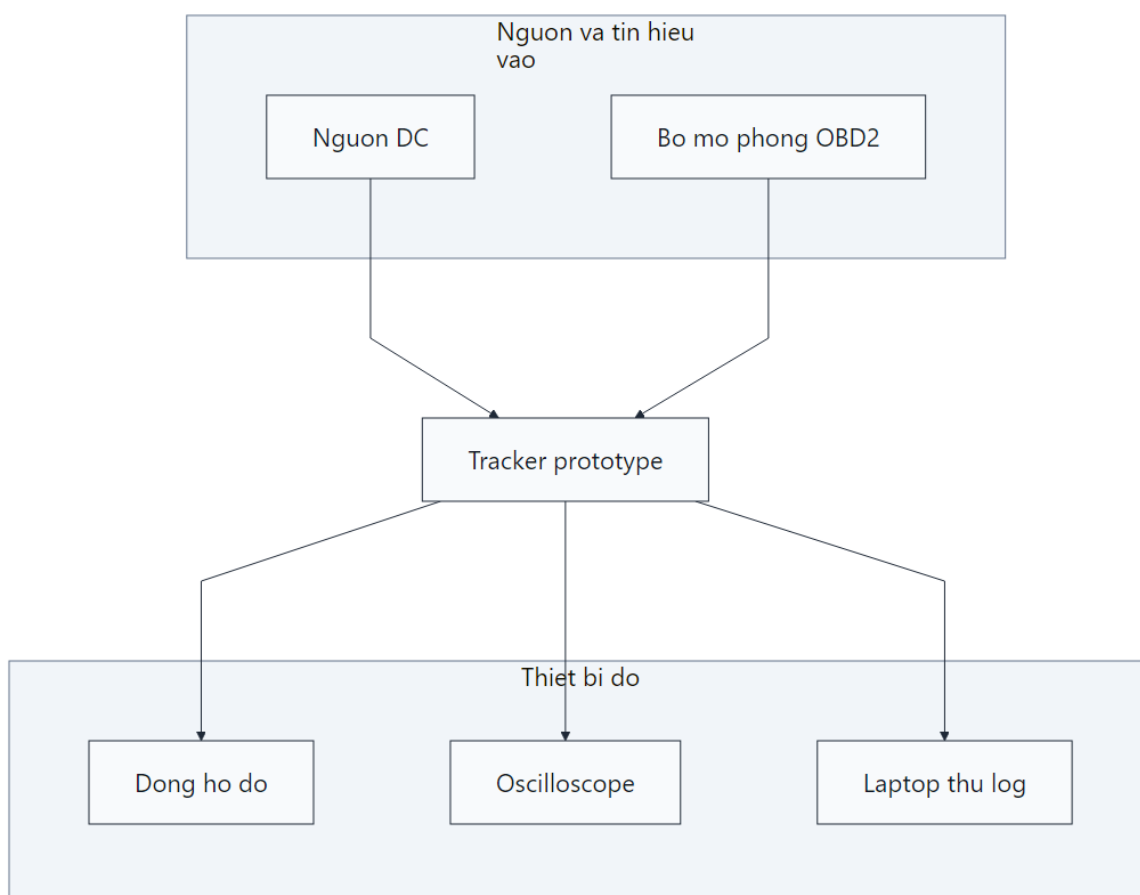
Hình 4.29: Bố trí thiết bị đo lường trong phòng thí nghiệm
