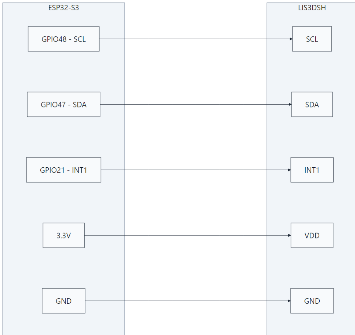
Hình 3.3: Sơ đồ kết nối LIS3DSH với ESP32-S3 qua I2C
