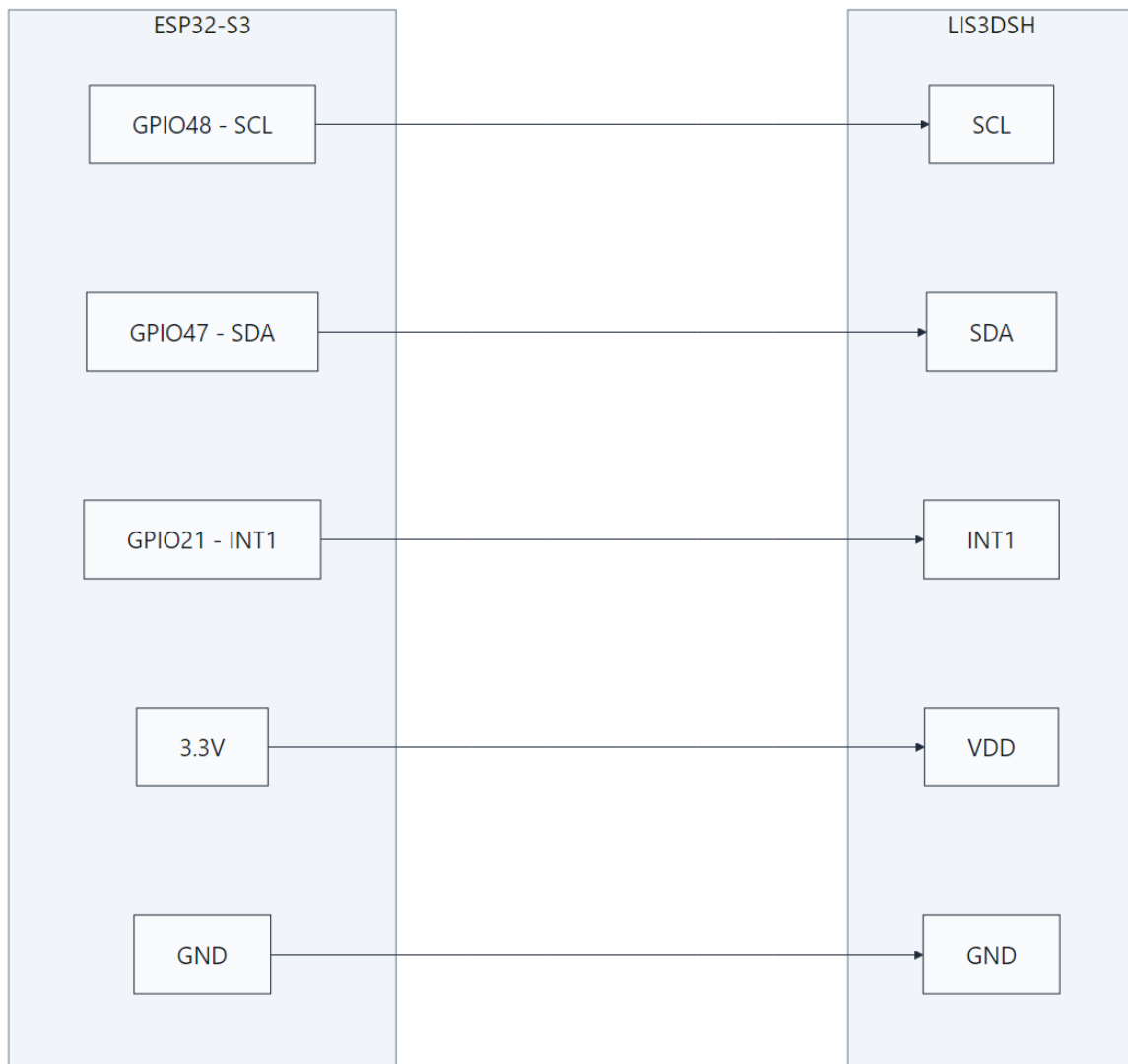
Hình 3.3a: Sơ đồ chi tiết chân kết nối LIS3DSH với ESP32-S3
