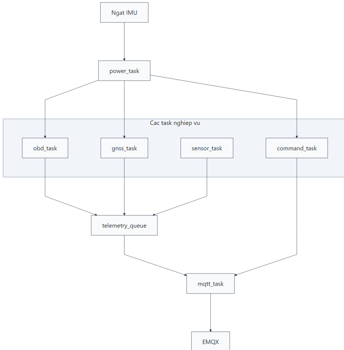
Hình 3.6: Sơ đồ tương tác giữa các FreeRTOS task
