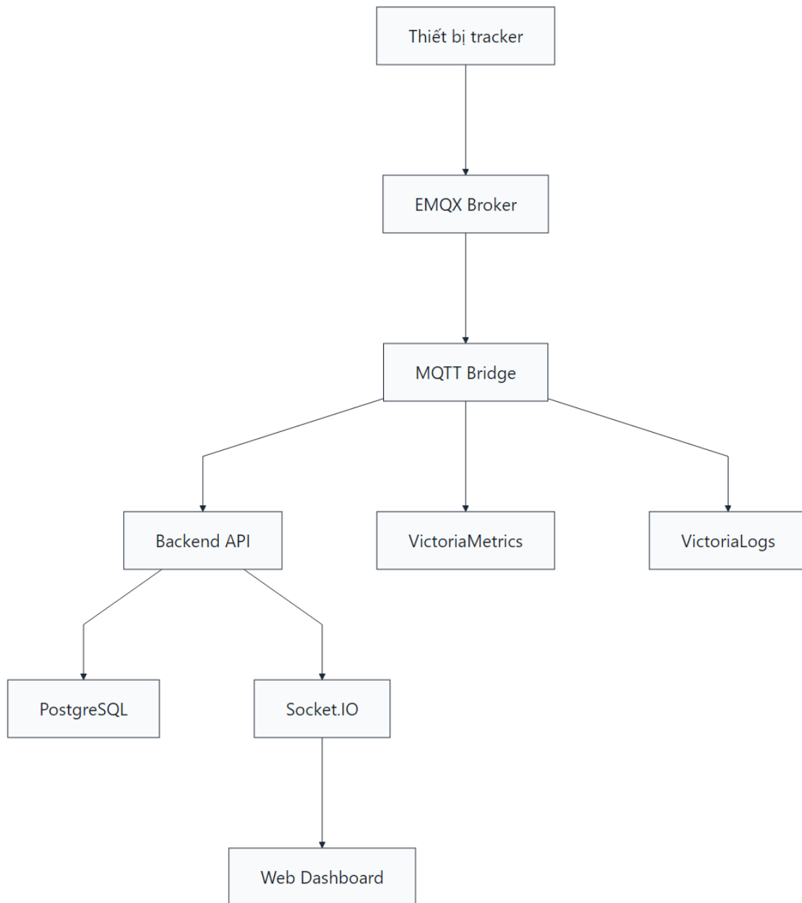
Hình 3.12: Sơ đồ kiến trúc tổng quan hệ thống Cloud
