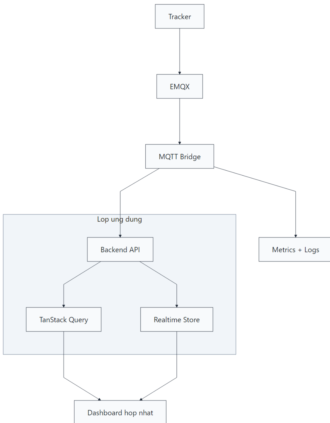
Hình 3.23: Sơ đồ kiến trúc tổng thể phương án tối ưu
