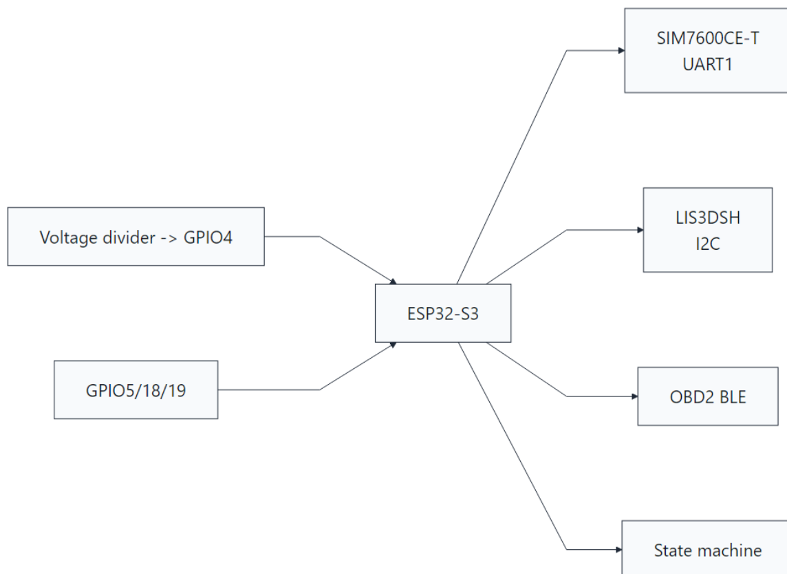
Hình 4.5: Sơ đồ đấu nối tổng thể giữa ESP32-S3 và các khối phần cứng tích hợp
