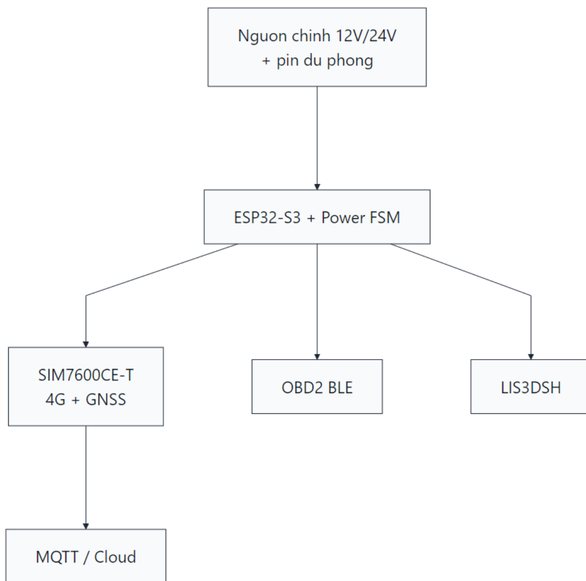
Hình 3.1: Sơ đồ khối tổng thể hệ thống tracker
