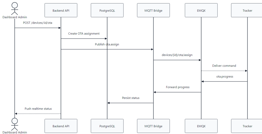
Hình 3.14a: Luồng điều phối OTA giữa Backend, EMQX, thiết bị và MQTT Bridge
