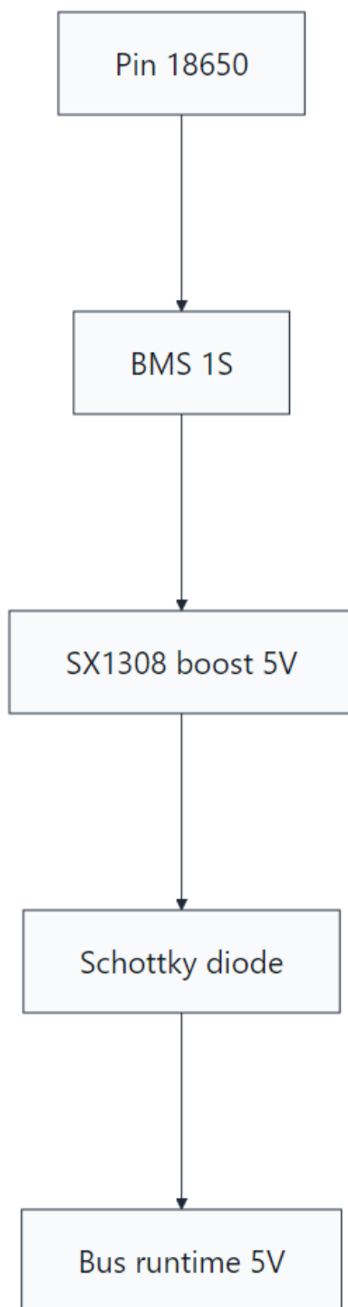
Hình 4.8: Kiến trúc nhánh nguồn dự phòng 5V từ pin 18650 qua SX1308
