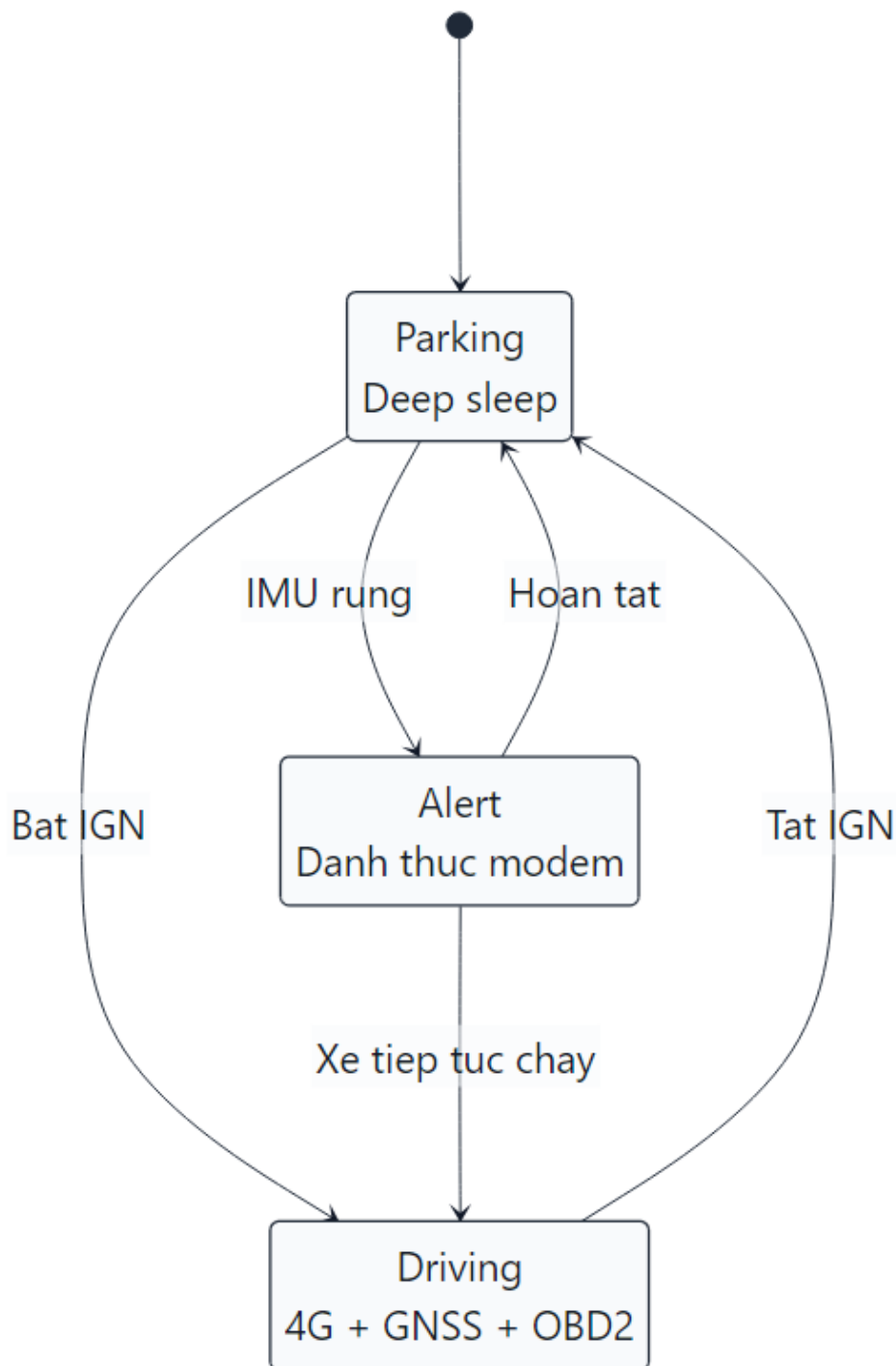
Hình 1.4: Sơ đồ chuyển đổi giữa các chế độ năng lượng
