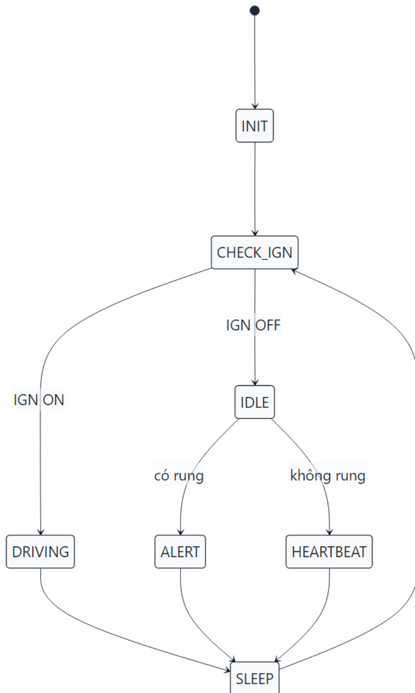
Hình 4.17: Lưu đồ thuật toán chính của firmware thiết bị theo dõi xe
