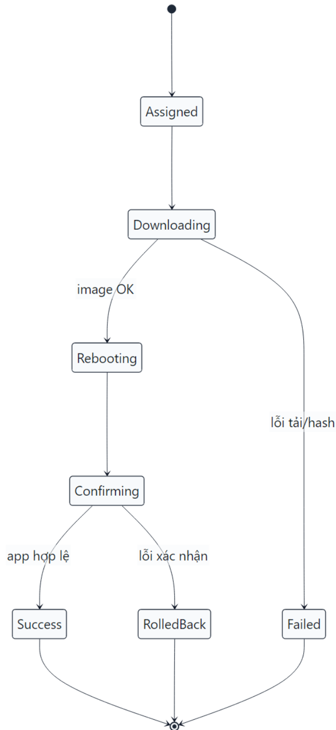
Hình 4.16a: Chuỗi bước OTA trên firmware từ nhận lệnh đến xác nhận sau reboot
