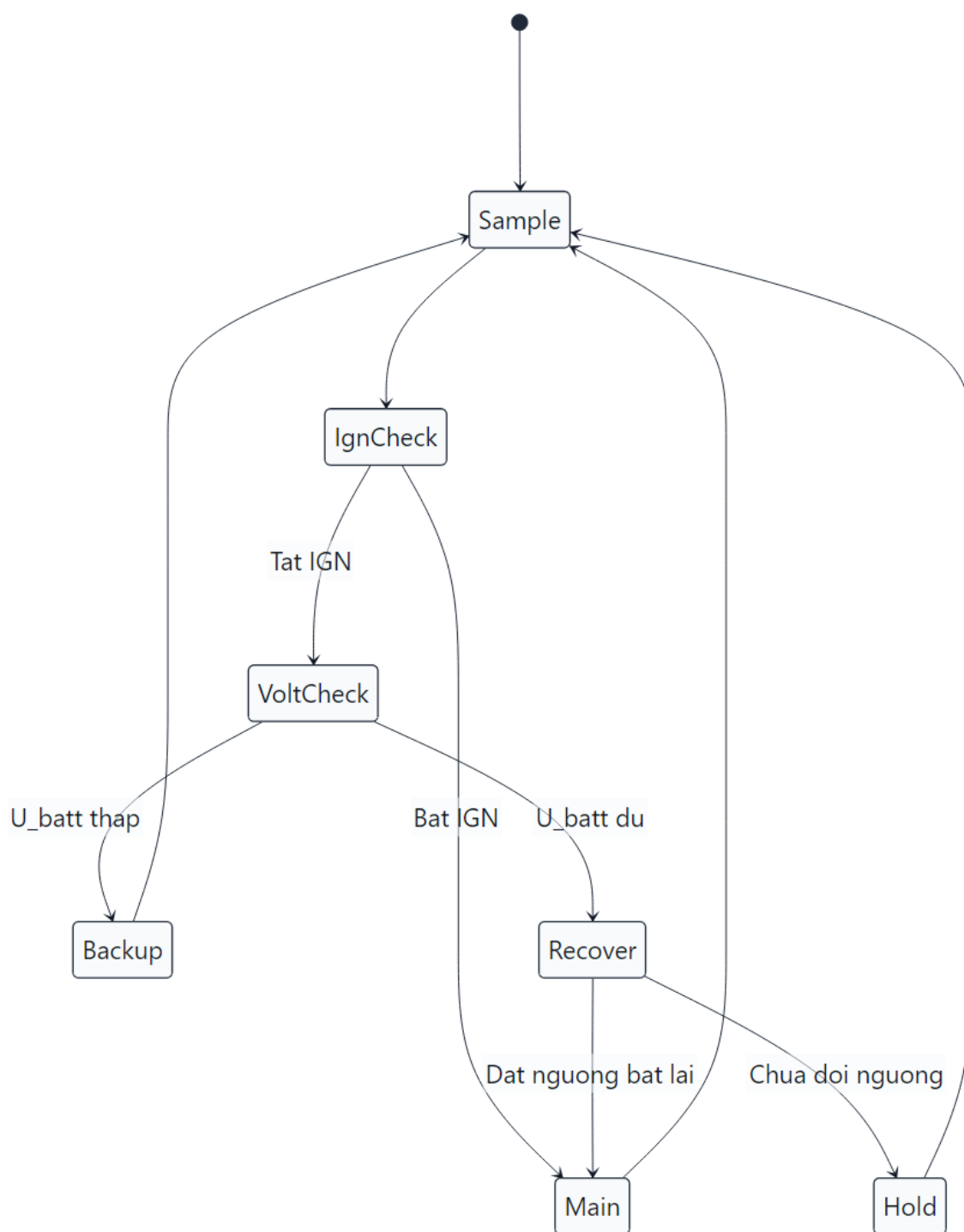
Hình 3.10: Lưu đồ thuật toán điều khiển power path
