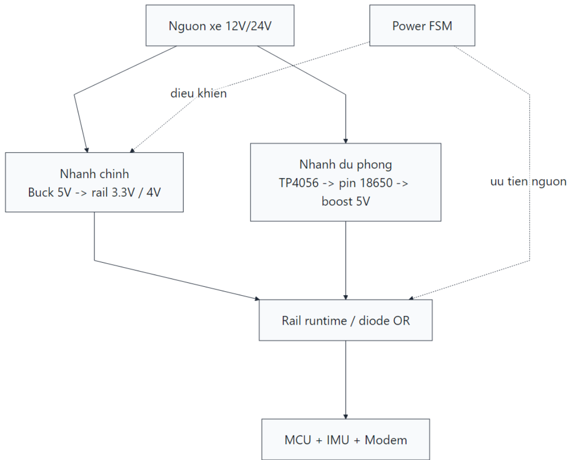
Hình 4.6: Kiến trúc tổng thể mạch quản lý nguồn
