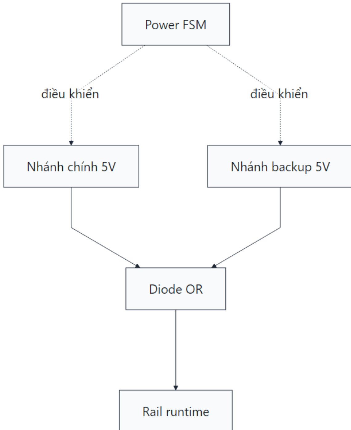
Hình 4.6a: Kiến trúc power path giữa nguồn xe và pin dự phòng
