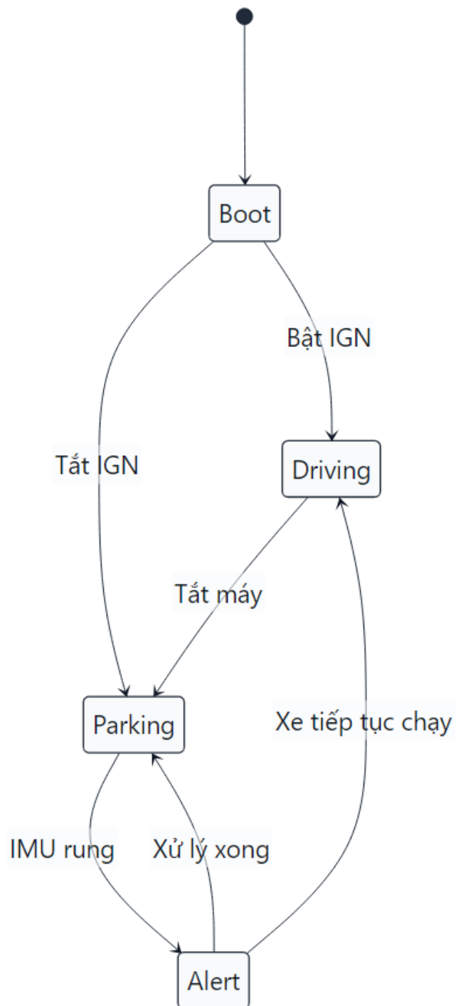
Hình 3.11: Sơ đồ máy trạng thái của thiết bị theo dõi
