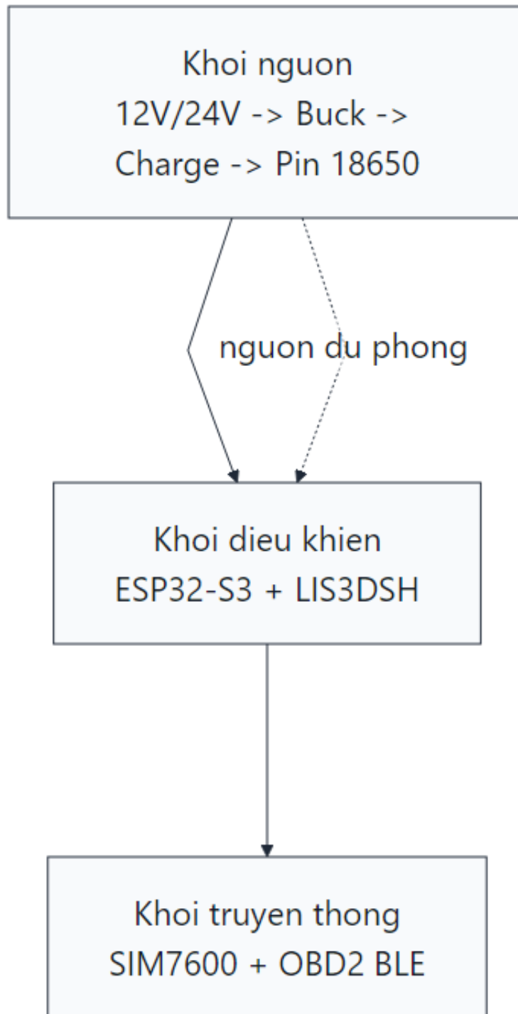
Hình 4.1a: Bố trí chi tiết các khối phần cứng trong tracker
