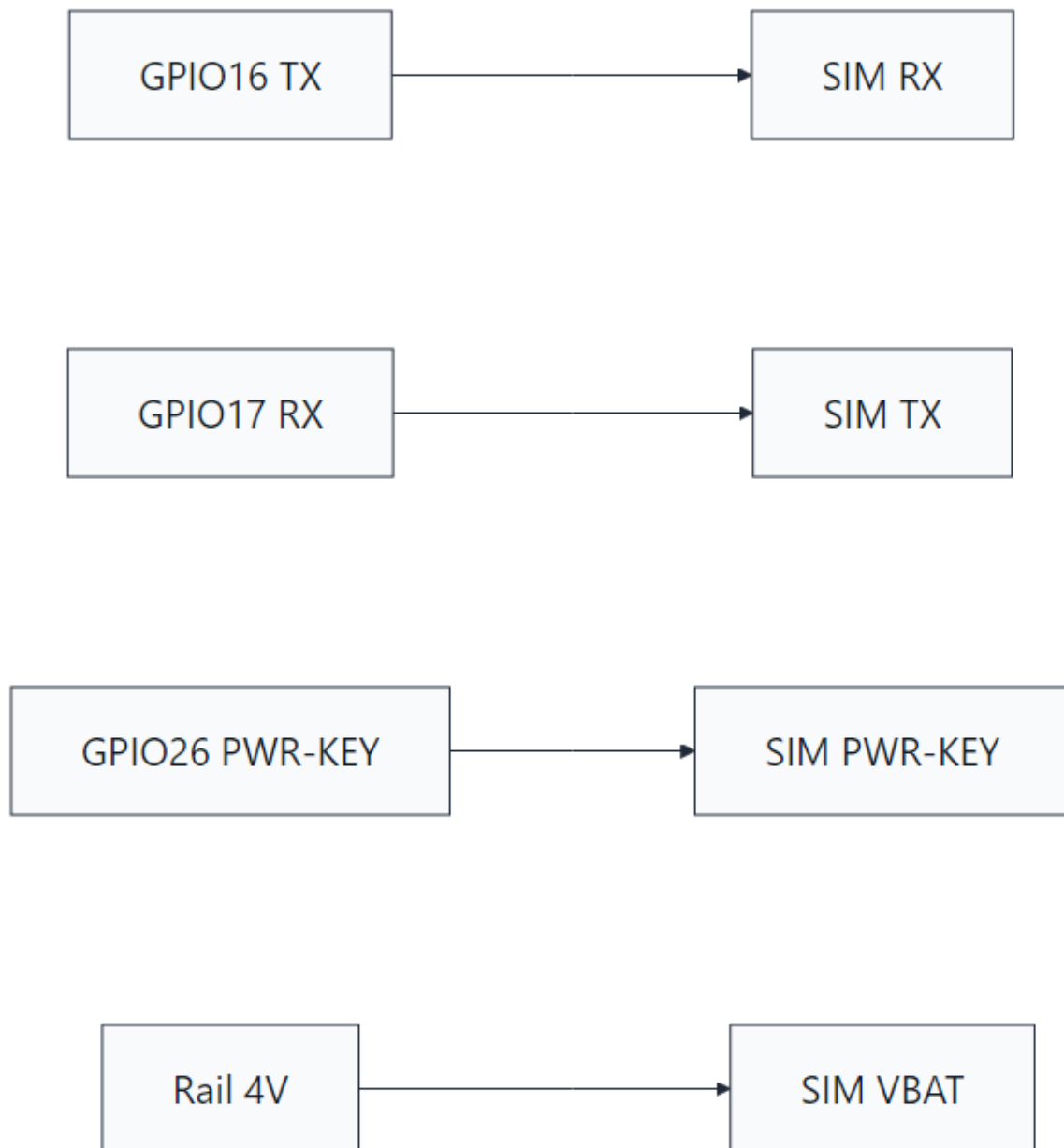
Hình 4.2: Sơ đồ kết nối giữa ESP32-S3 và modem SIM7600CE-T qua UART
