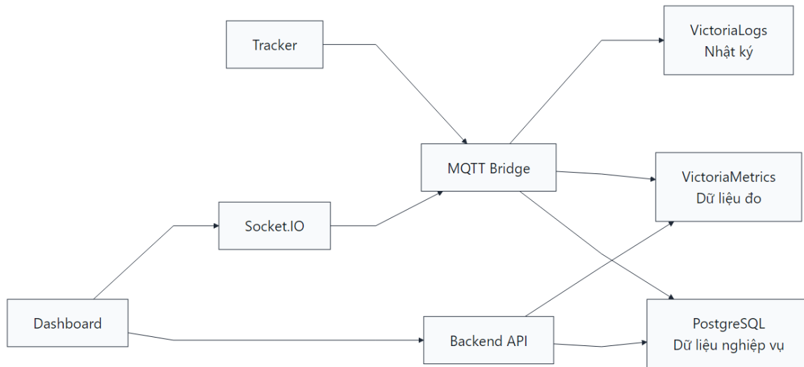
Hình 2.1: Sơ đồ kiến trúc dữ liệu của hệ thống - Data Architecture Diagram
