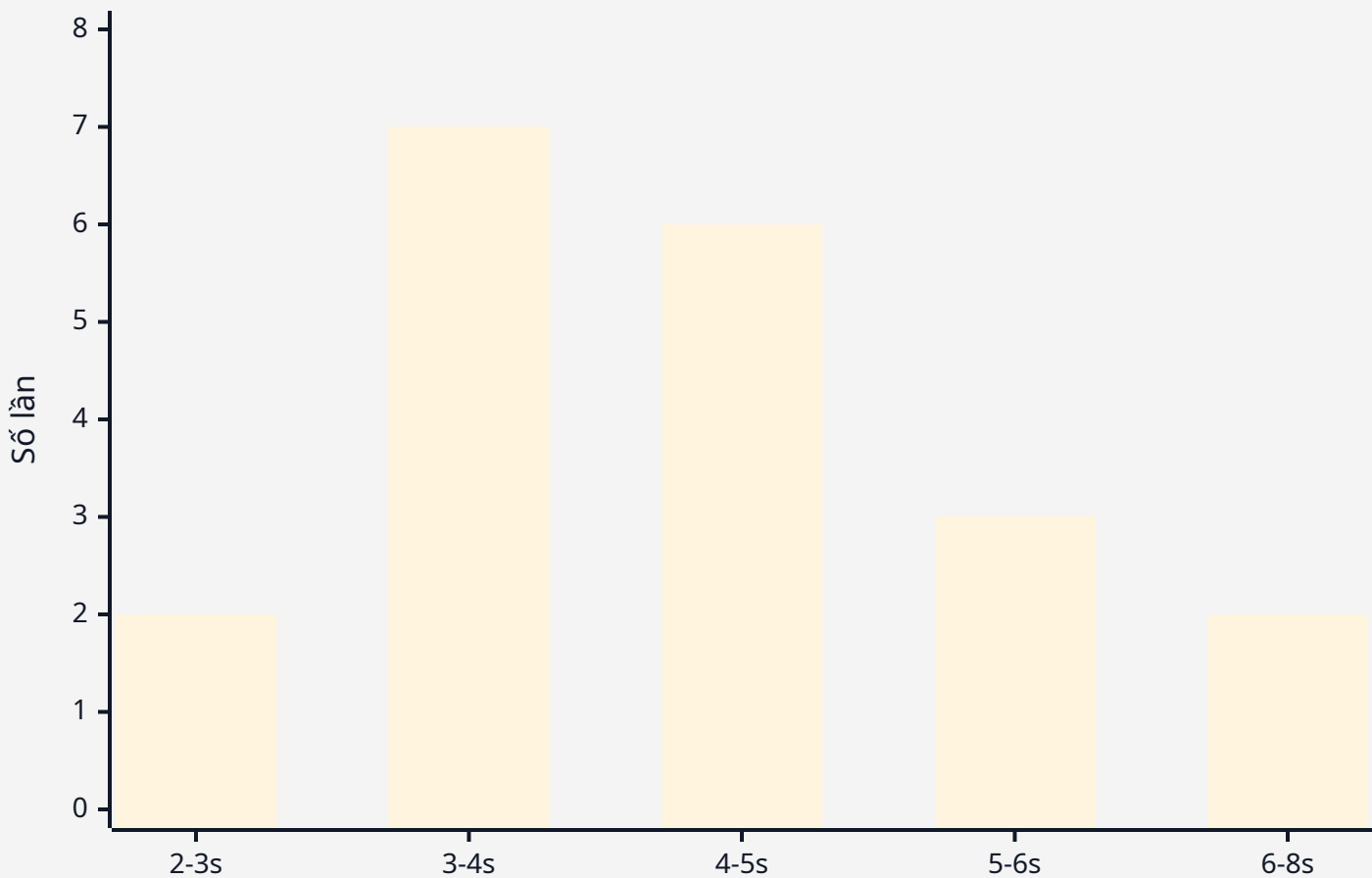
Phân bố thời gian kết nối OBD2 BLE
