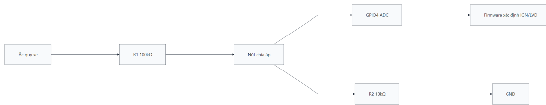
Hình 4.3: Sơ đồ mạch đo điện áp ắc quy bằng voltage divider và ADC ESP32-S3
