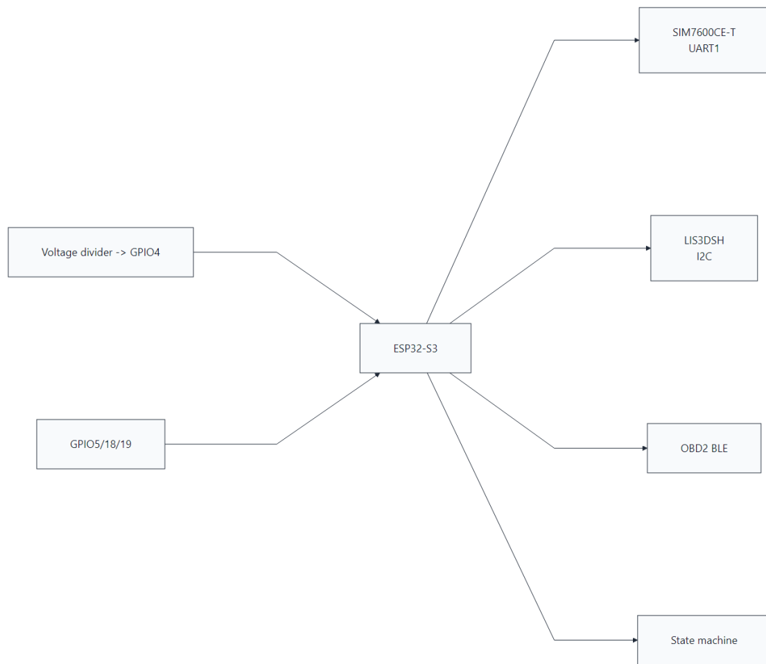
Hình 4.5: Sơ đồ đầu nối tổng thể giữa ESP32-S3 và các khối phần cứng tích hợp
