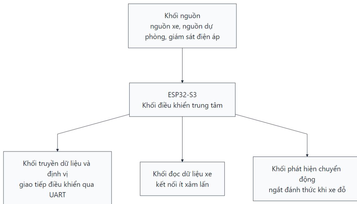
Hình 3.2: Phân rã các khối phần cứng chính xoay quanh ESP32-S3
