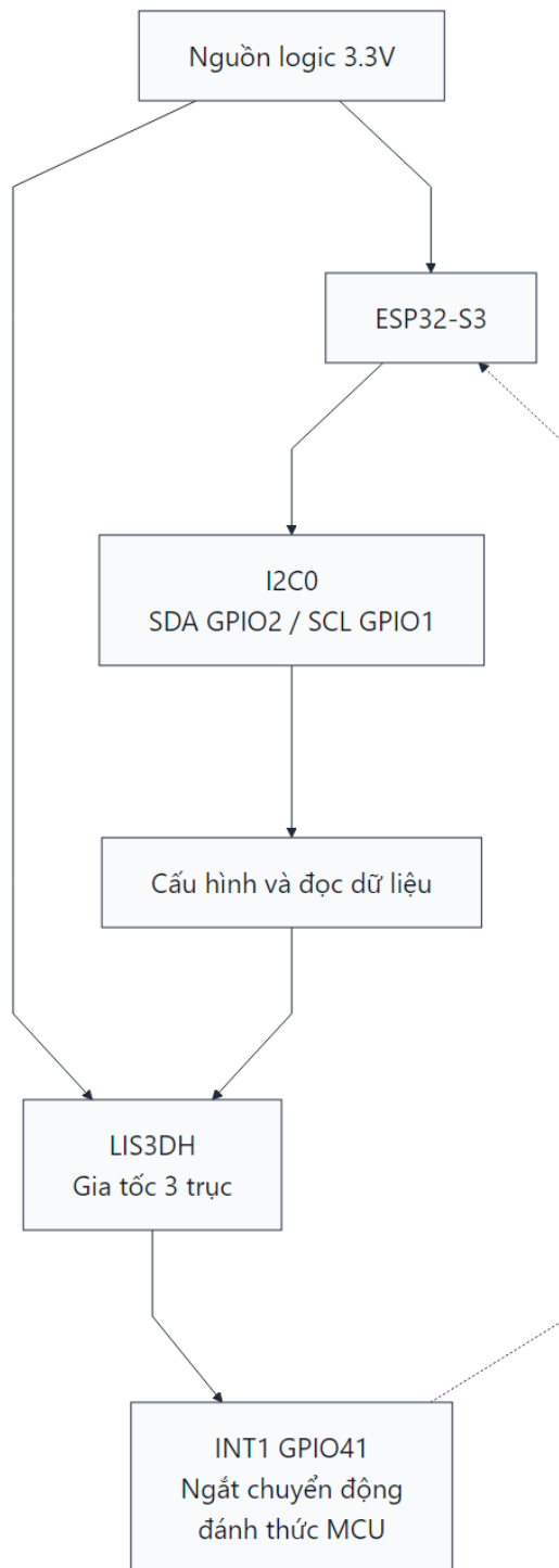
Hình 3.5: Cảm biến LIS3DH và kết nối I2C/ngắt với ESP32-S3
