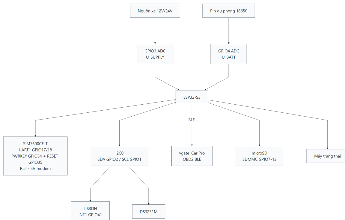
Hình 4.1: Sơ đồ đấu nối tổng thể giữa ESP32-S3 và các khối phần cứng tích hợp
