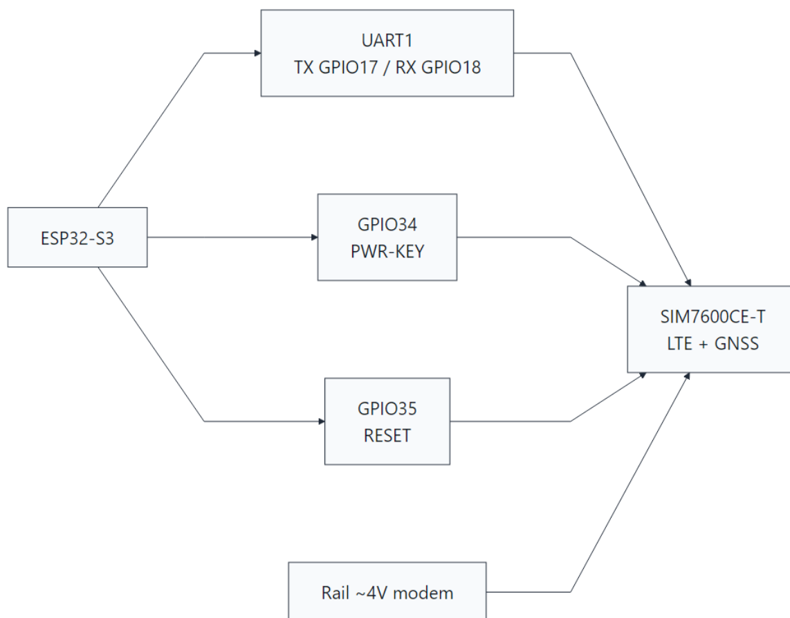
Hình 3.3: Kết nối UART giữa ESP32-S3 và mô-đun SIM7600CE-T
