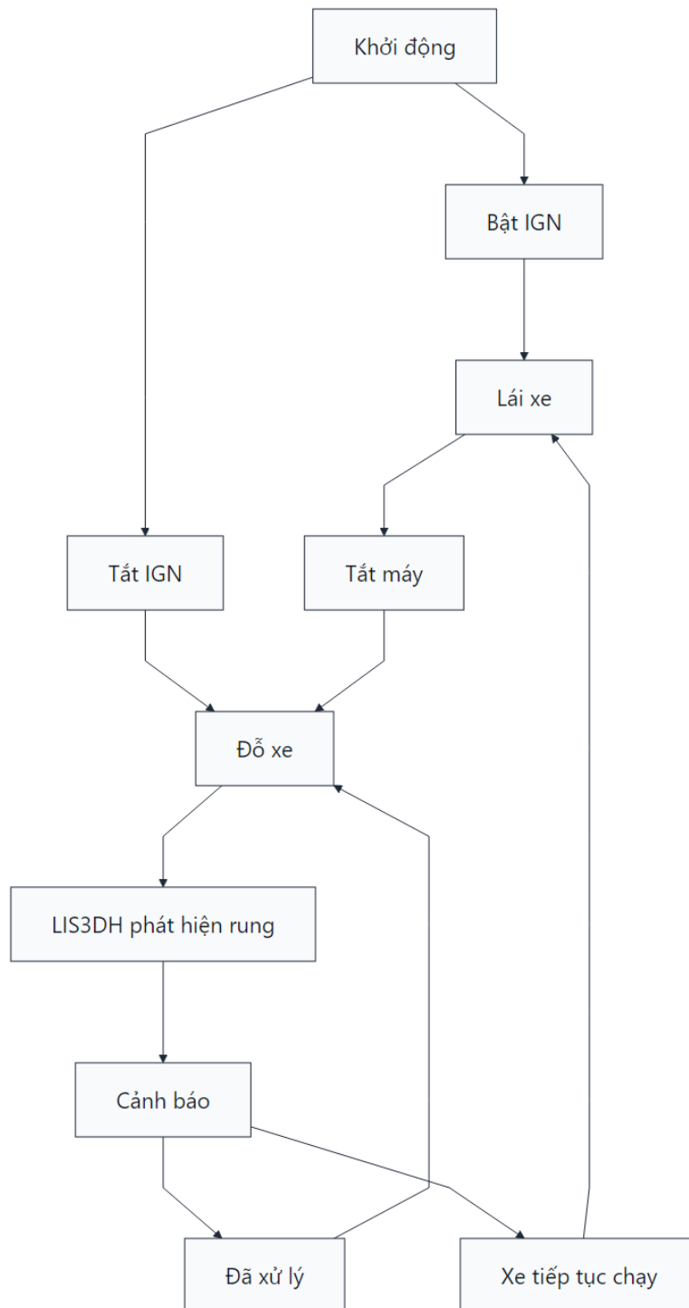
Hình 3.7: Sơ đồ máy trạng thái vận hành chính của firmware
