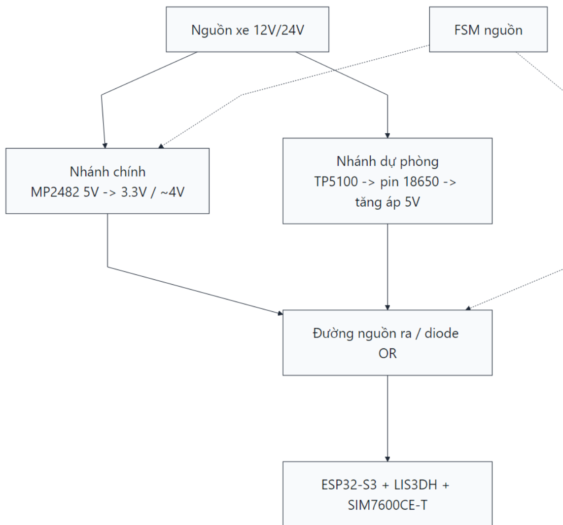
Hình 3.6: Sơ đồ khối hệ thống quản lý nguồn của thiết bị
