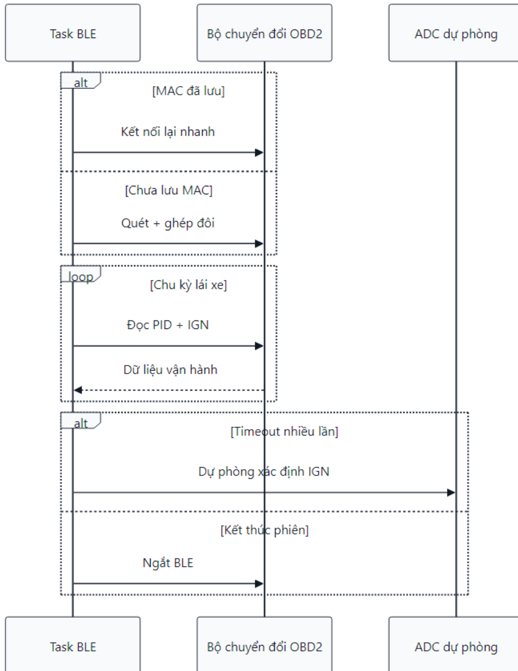
Hình 3.8: Luồng kết nối và đọc dữ liệu BLE OBD2 trong firmware
