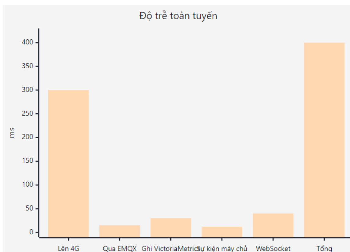
Hình 4.39: Đồ thị phân bố độ trễ toàn tuyến (1000 bản tin mẫu)
