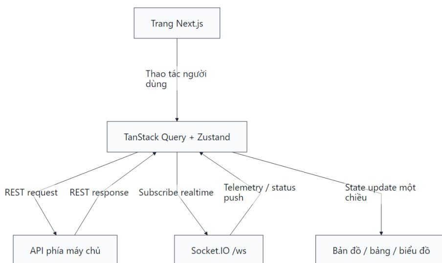
Hình 3.15a: Luồng dữ liệu một chiều giữa Next.js, Query, Zustand và API máy chủ
