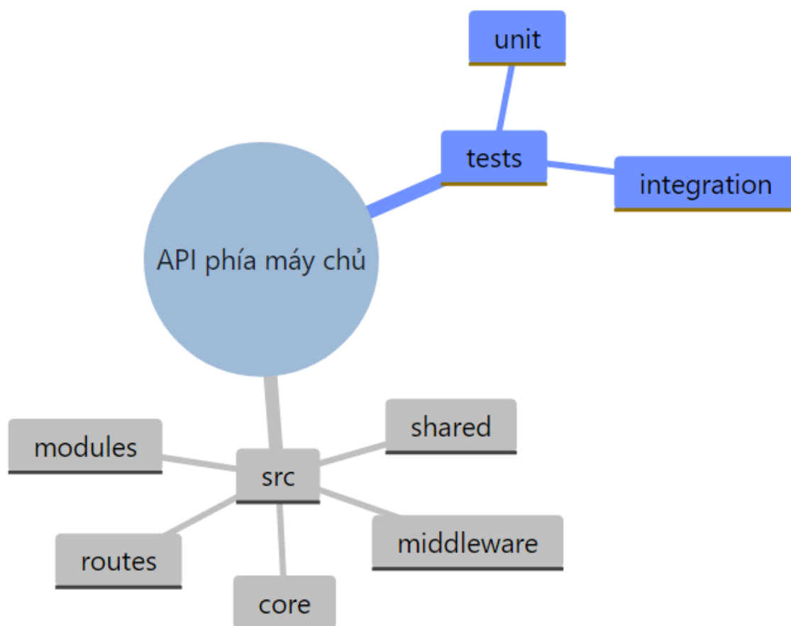
Hình 4.21: Cấu trúc thư mục API máy chủ theo kiến trúc DDD
