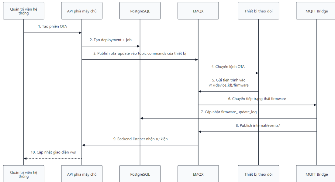
Hình 3.14a: Luồng điều phối OTA giữa API máy chủ, EMQX, thiết bị và MQTT Bridge
