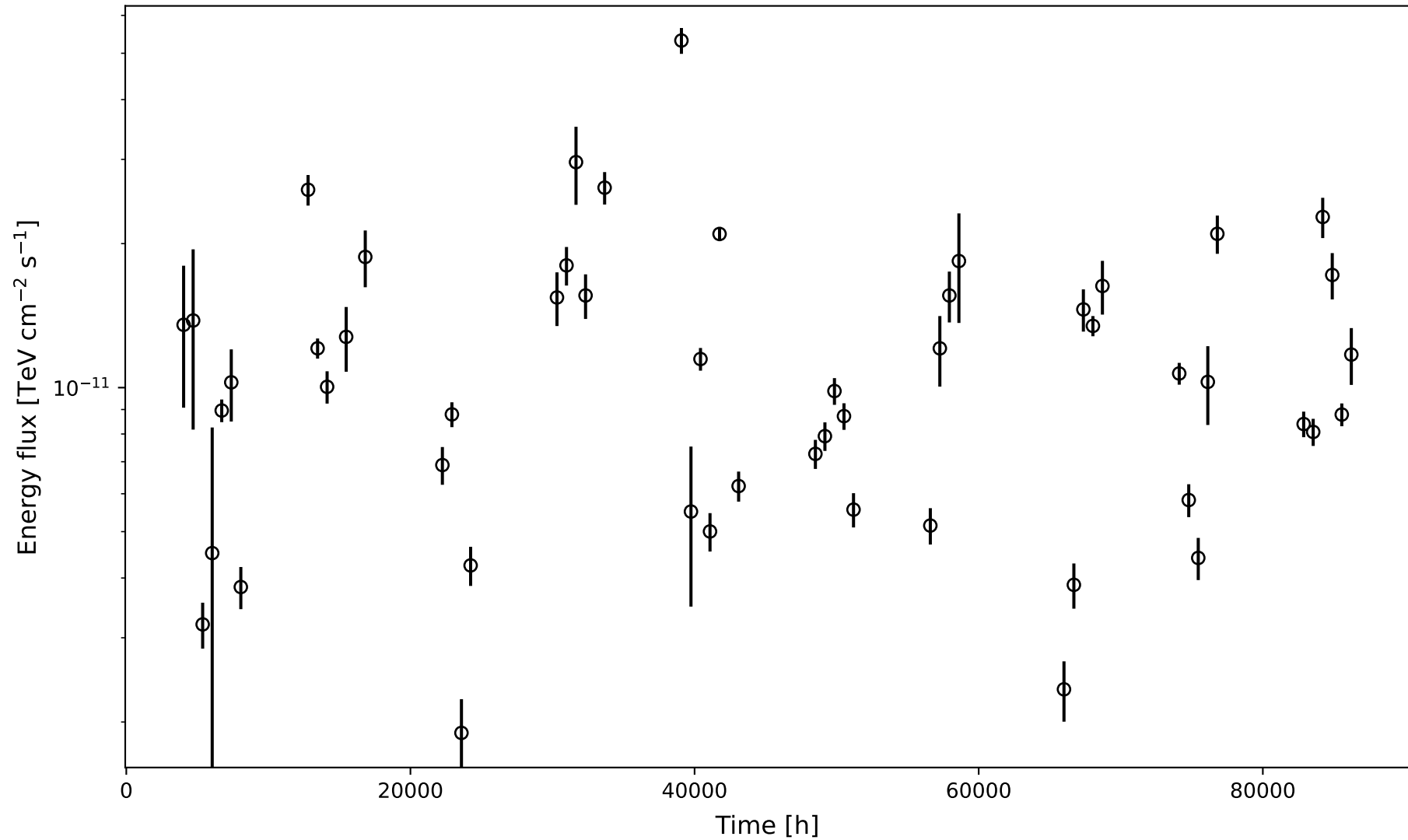
BLLac_check_100_120min - CTAO simulation
