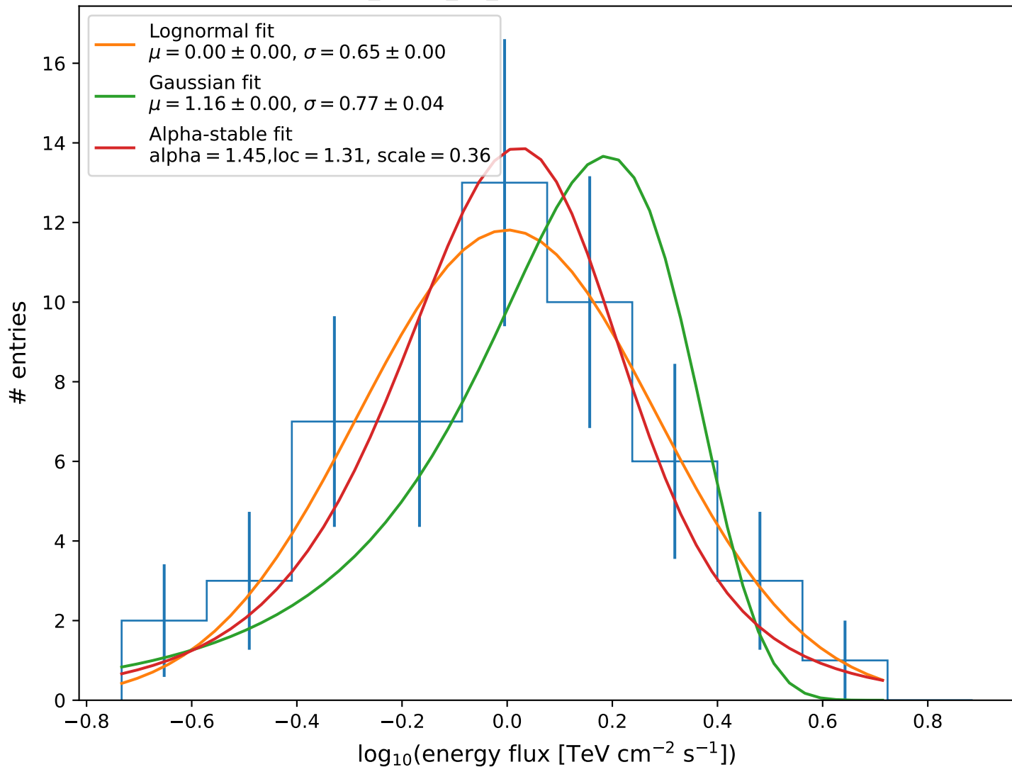
BLLac_check_10_120min - CTAO simulation
