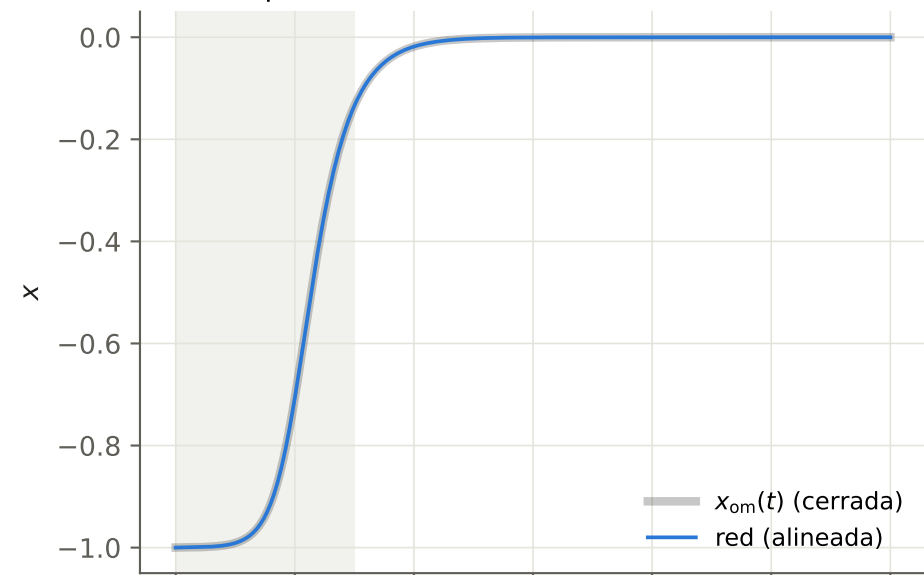
A.1 escape térmico (S·D)
