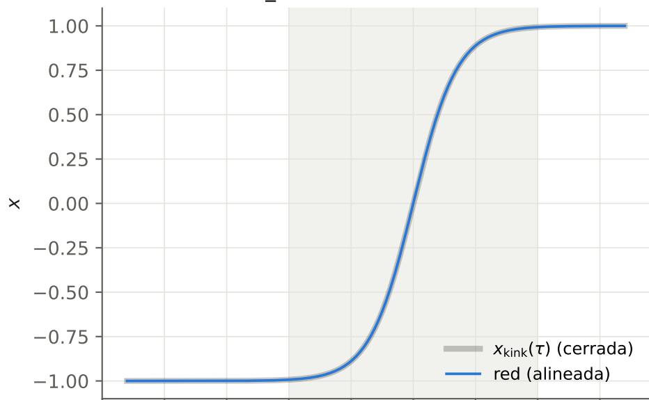
A.2 instantón (S_E)
