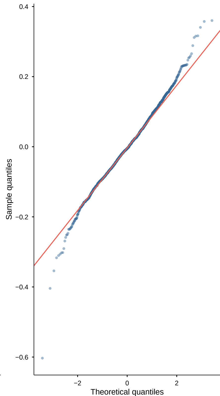
C Q-Q
