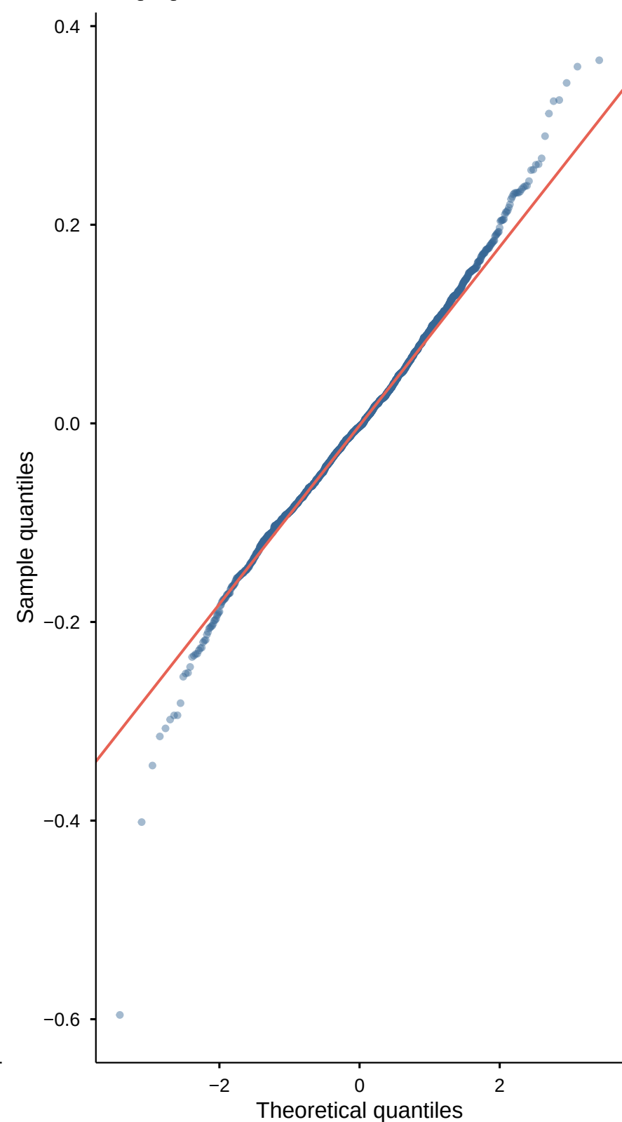
C Q-Q
