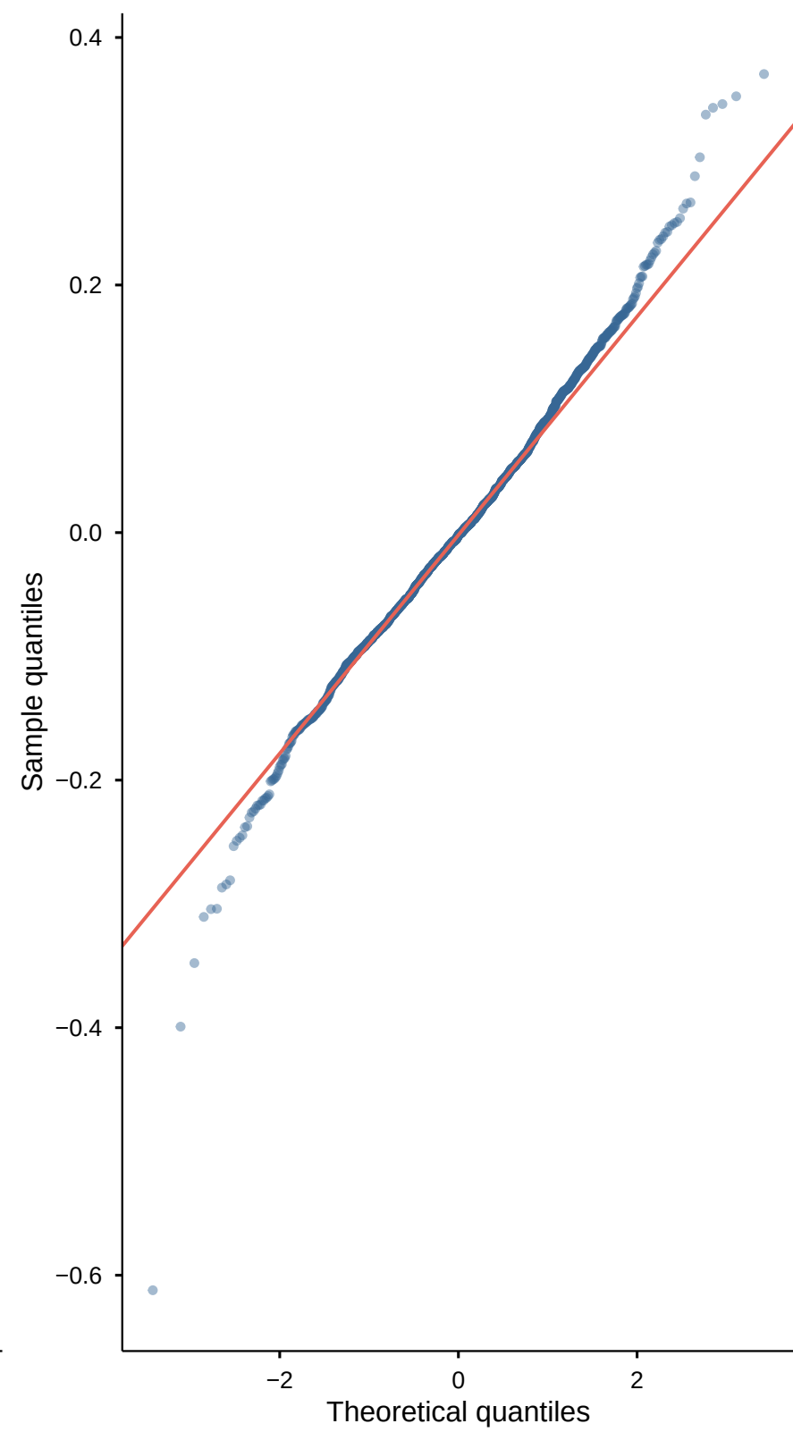
C Q-Q
