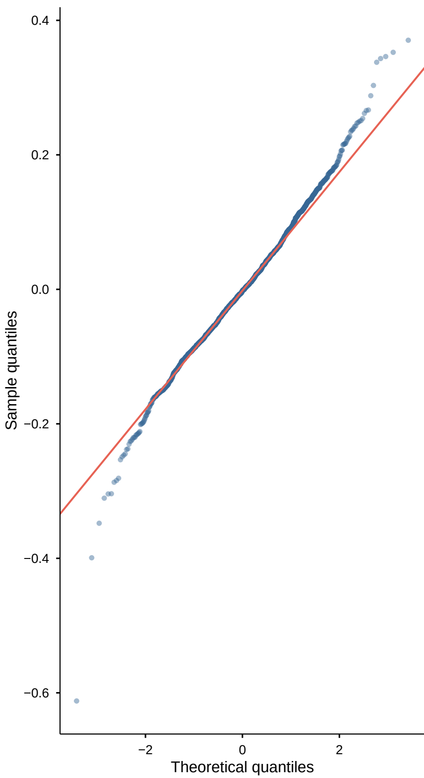
C Q-Q
