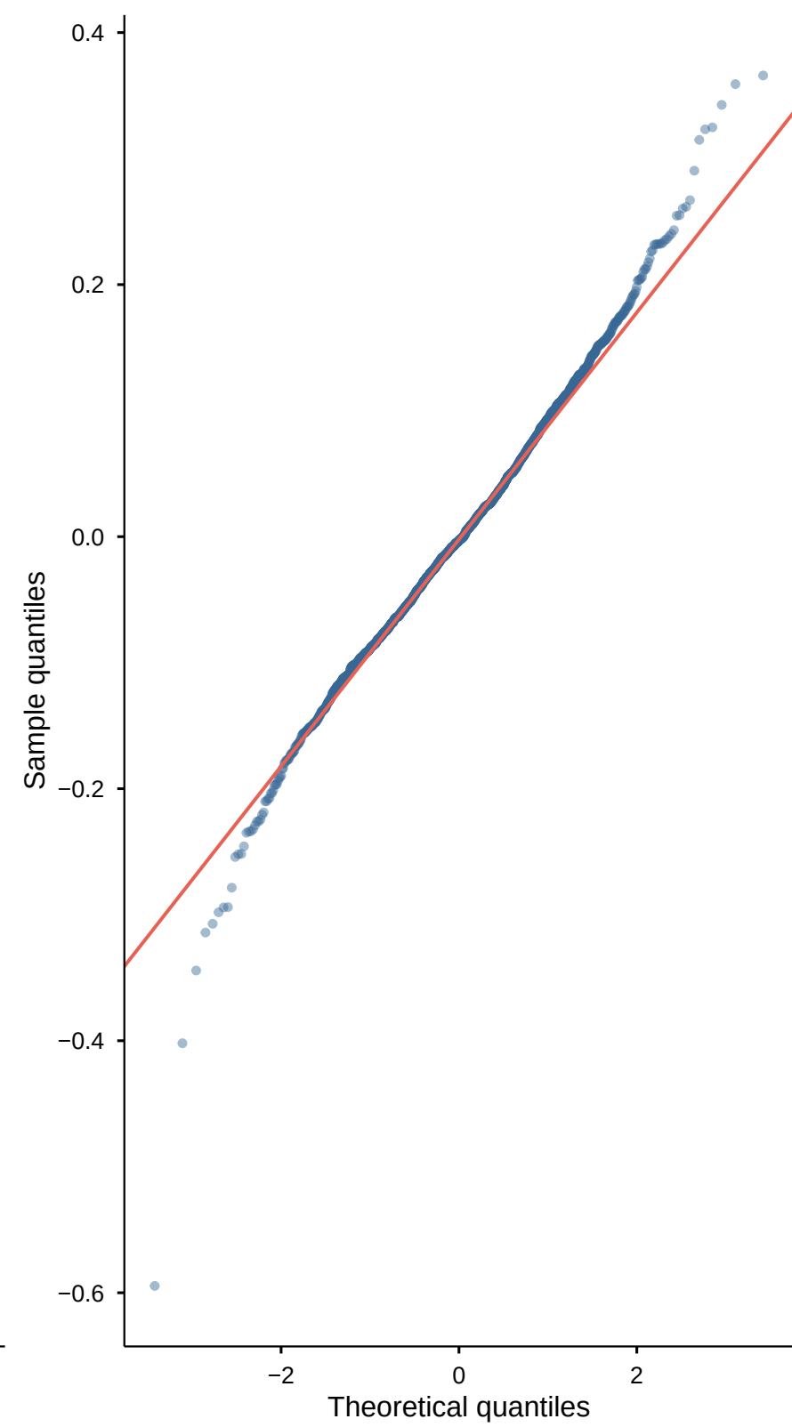
C Q-Q
