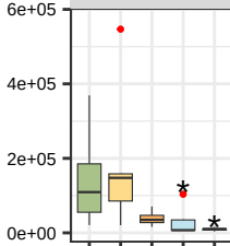
Vestitol (F932)
