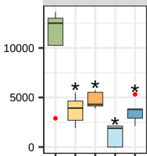
Naringenin (F928)
