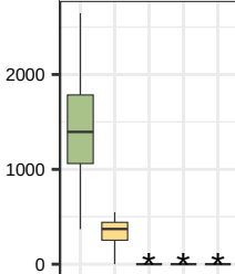
Gibberellin (F2320)
