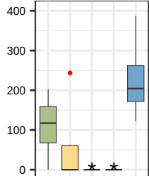
Esculetin (F494)
