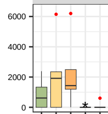
Buxuletin/Scopoletin (F439)
