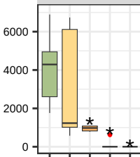
Quercetin (F1783)
