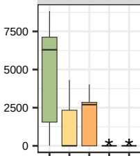
Diosmetin (F1130)
