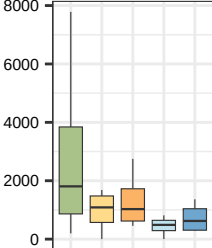
Saponarin (F3287)
