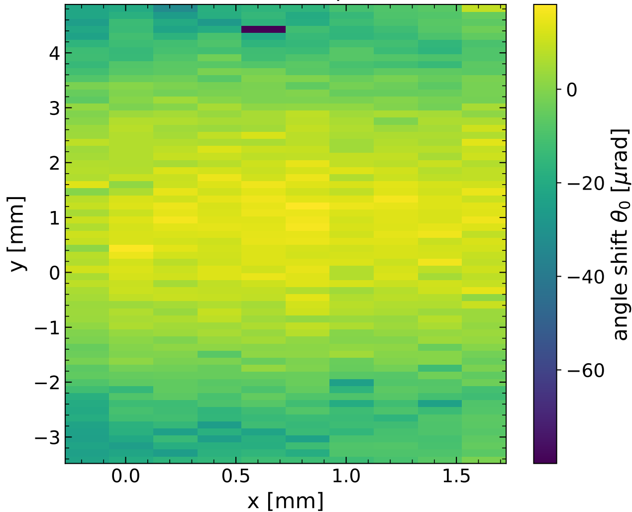
Torsion Map
