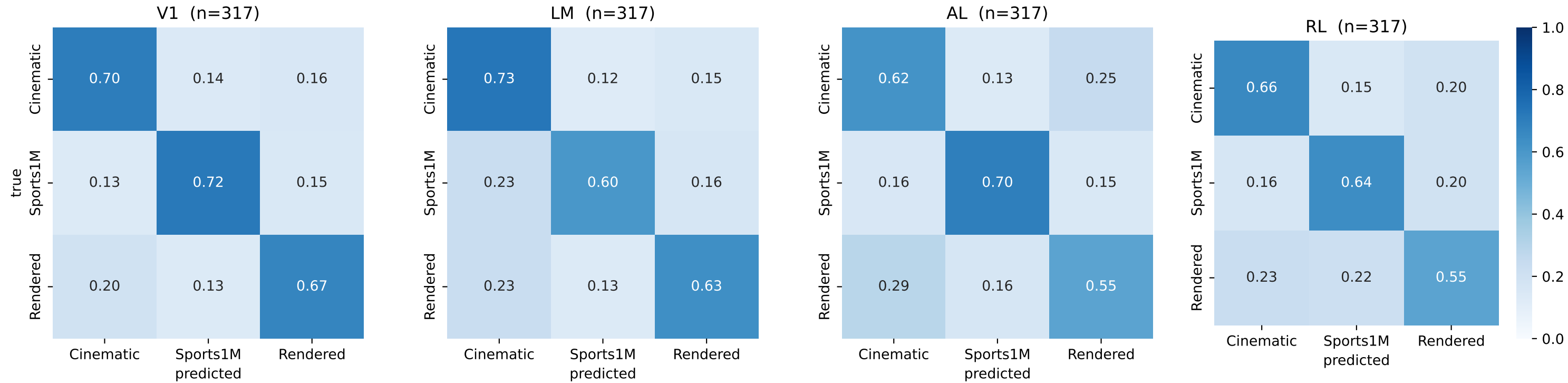
Q1c confusion matrices — session 6_4
