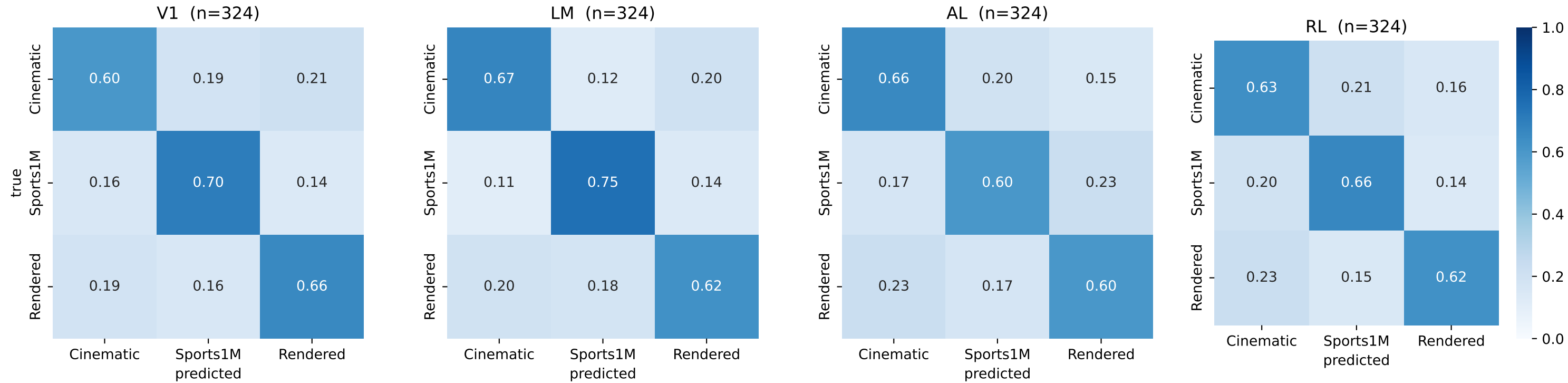
Q1c confusion matrices — session 7_3
