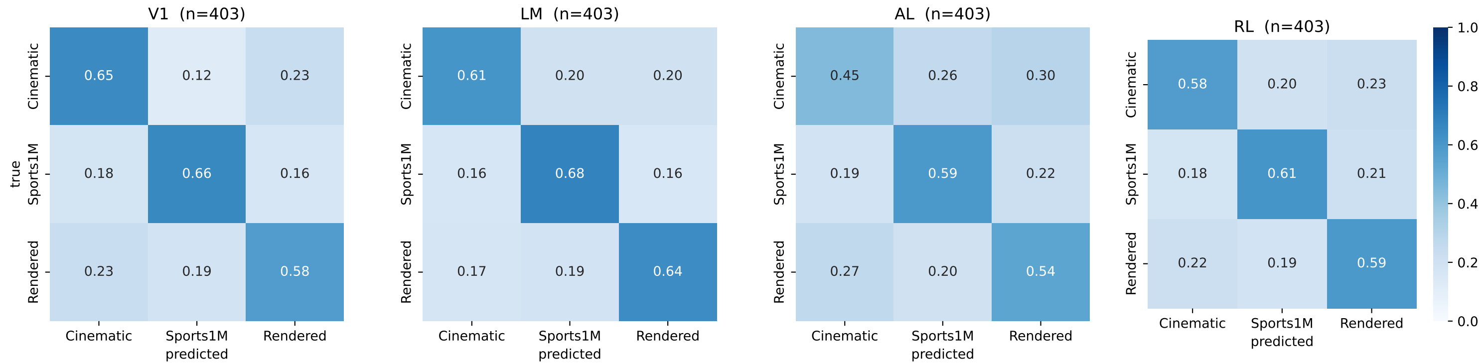
Q1c confusion matrices — session 5_7
