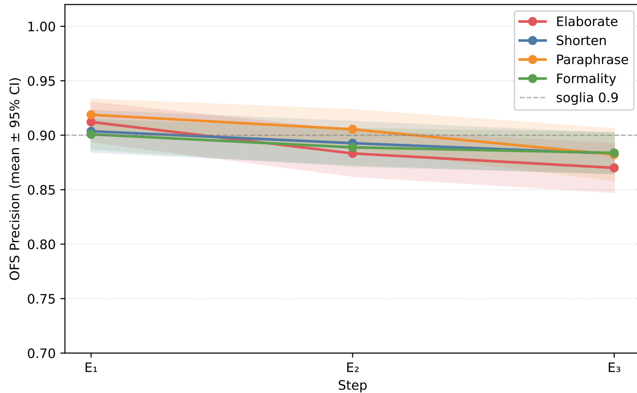
OFS Precision — 25 qid
