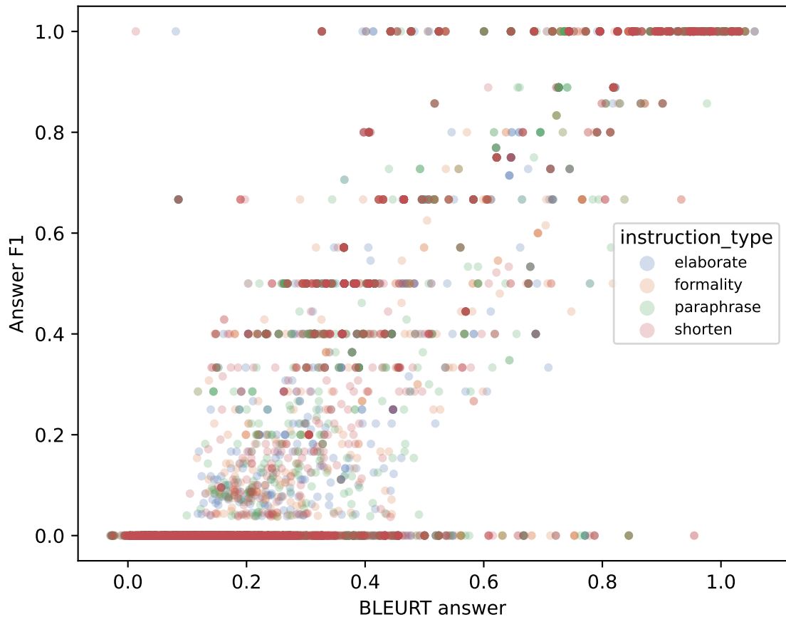
BLEURT answer vs Answer F1
