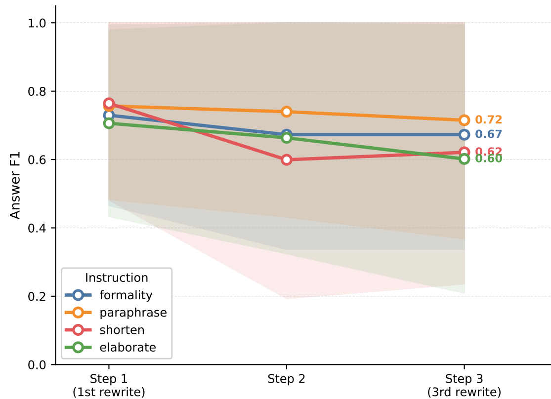
Answer F1
