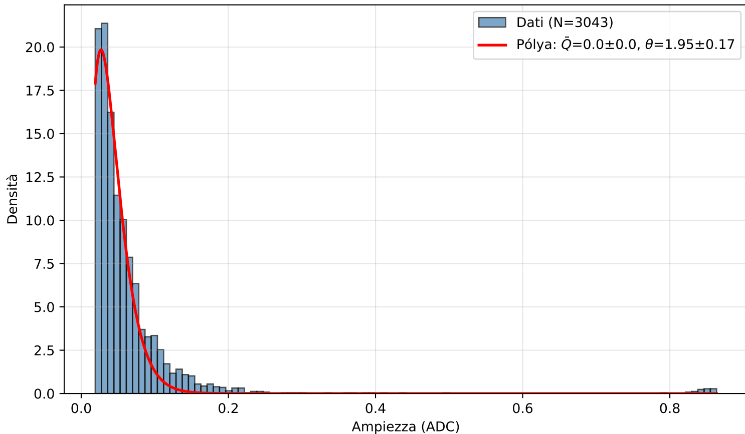
PICOSEC Detector 1 — Canale (5.0, 3.0)
