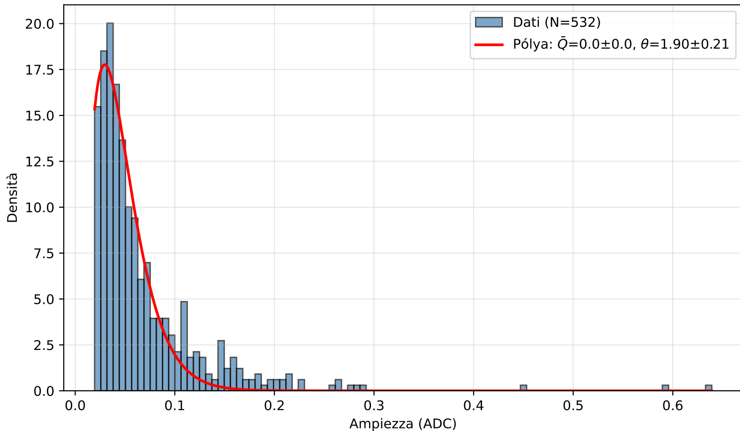
PICOSEC Detector 1 — Canale (7.0, 5.0)
