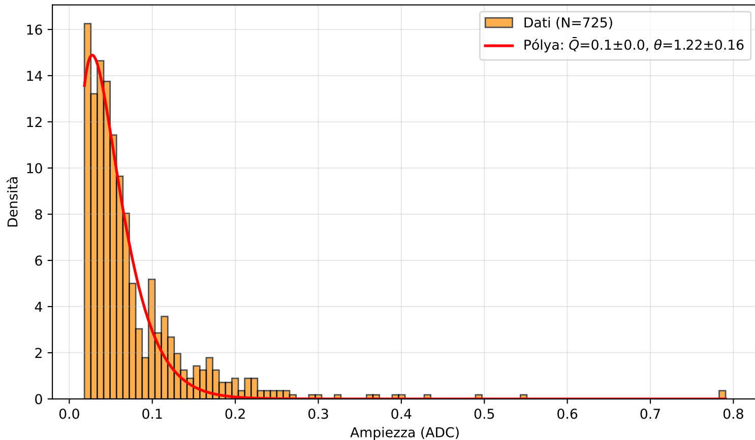
PICOSEC Detector 2 — Canale (3.0, 8.0)
