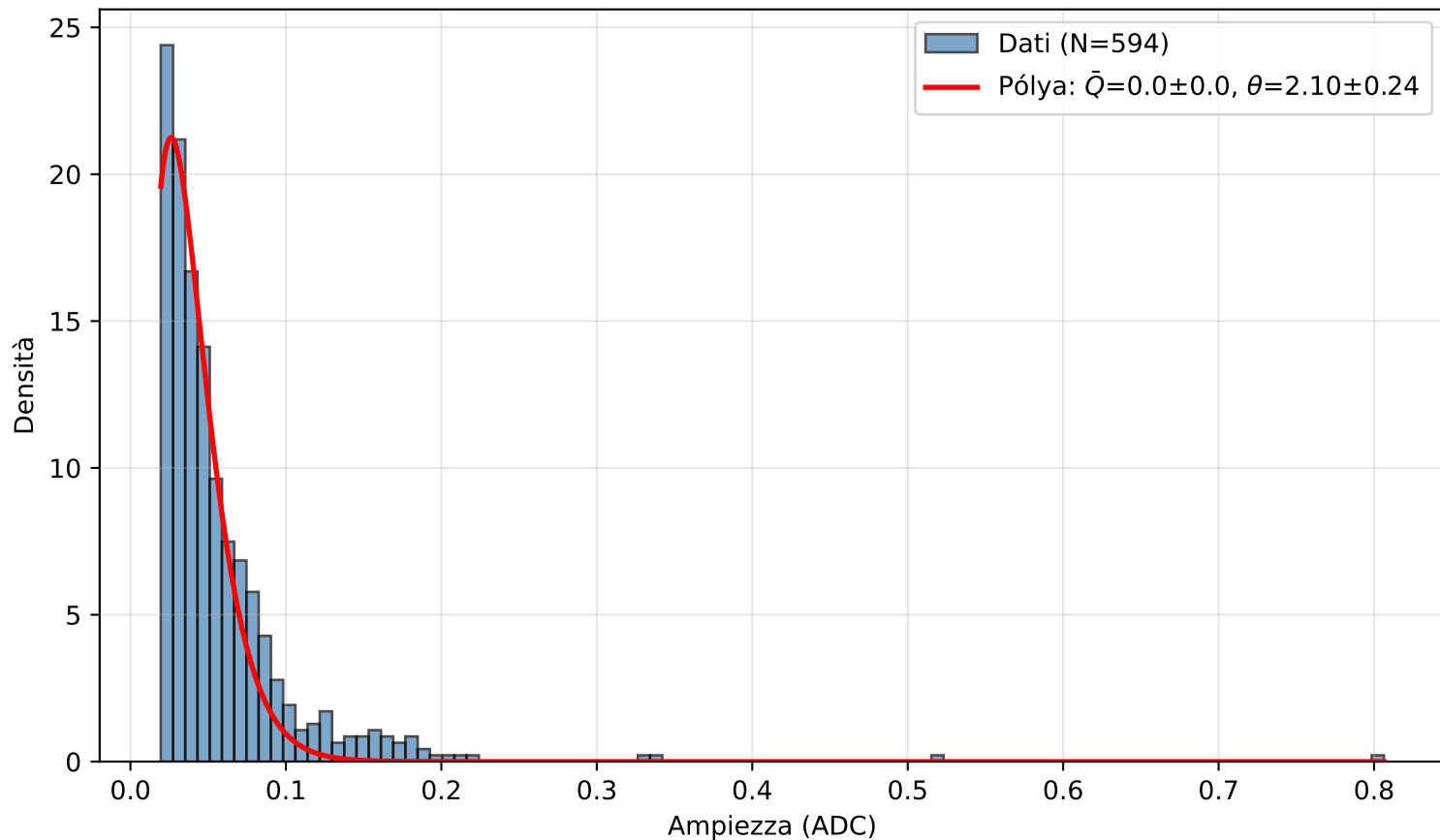
PICOSEC Detector 1 — Canale (7.0, 6.0)
