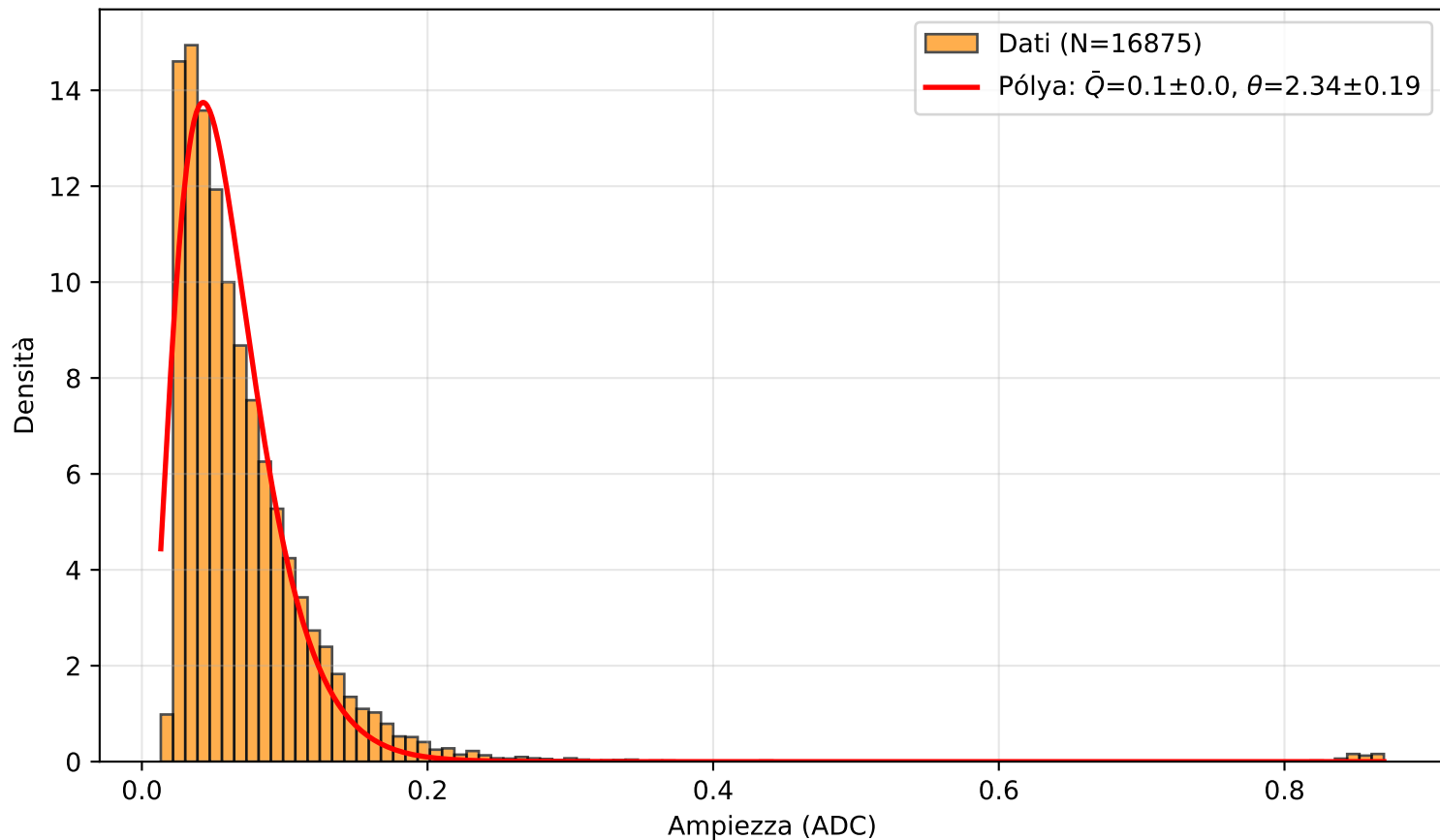
PICOSEC Detector 2 — Canale (5.0, 6.0)
