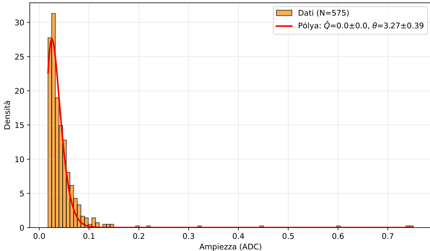
PICOSEC Detector 2 — Canale (1.0, 2.0)
