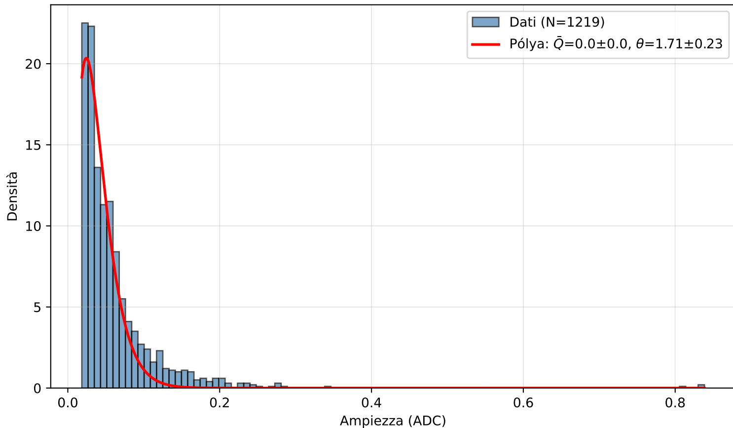
PICOSEC Detector 1 — Canale (3.0, 2.0)
