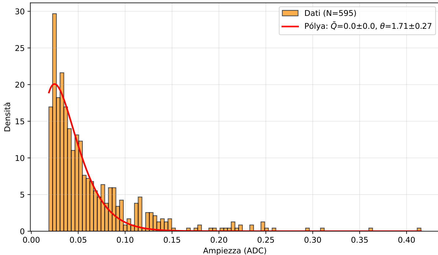
PICOSEC Detector 2 — Canale (8.0, 0.0)
