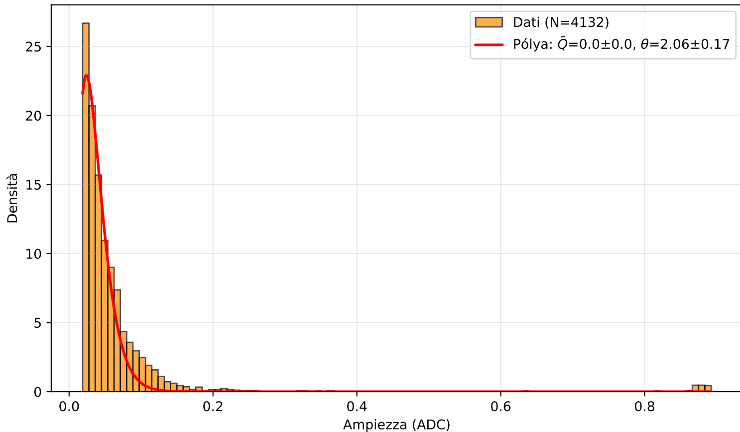
PICOSEC Detector 2 — Canale (4.0, 3.0)
