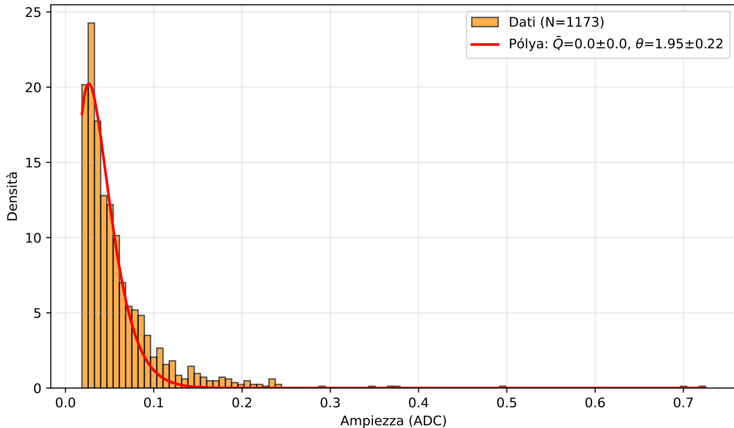
PICOSEC Detector 2 — Canale (6.0, 2.0)
