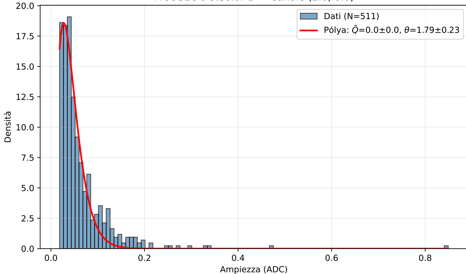
PICOSEC Detector 1 — Canale (2.0, 6.0)
