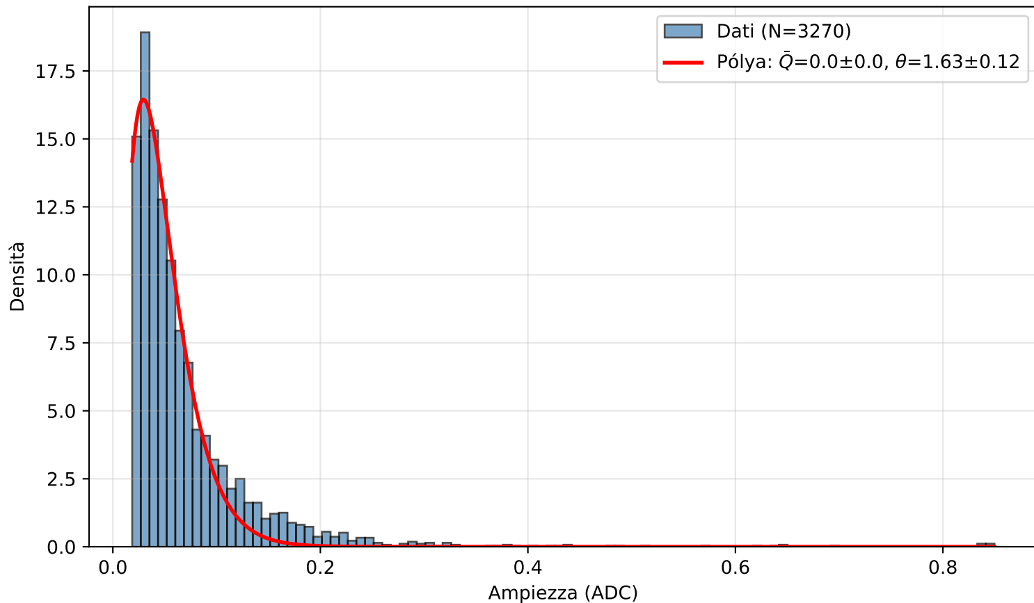
PICOSEC Detector 1 — Canale (4.0, 6.0)
