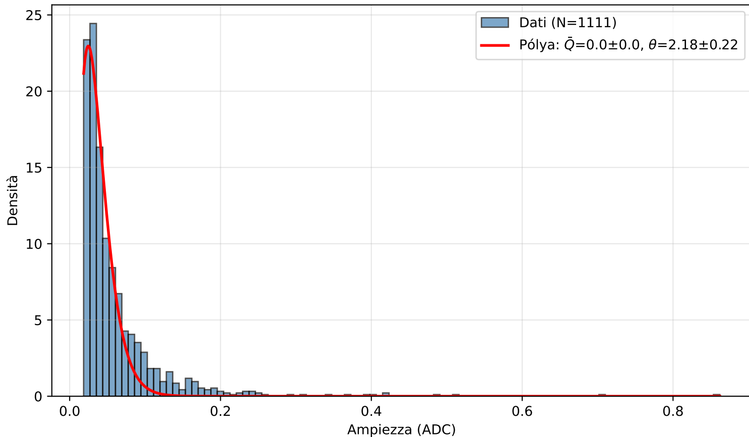
PICOSEC Detector 1 — Canale (4.0, 7.0)
