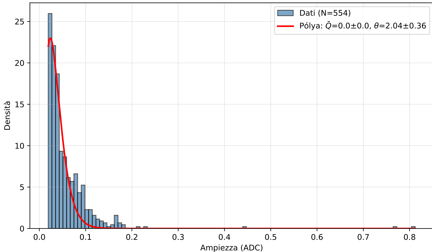
PICOSEC Detector 1 — Canale (7.0, 7.0)
