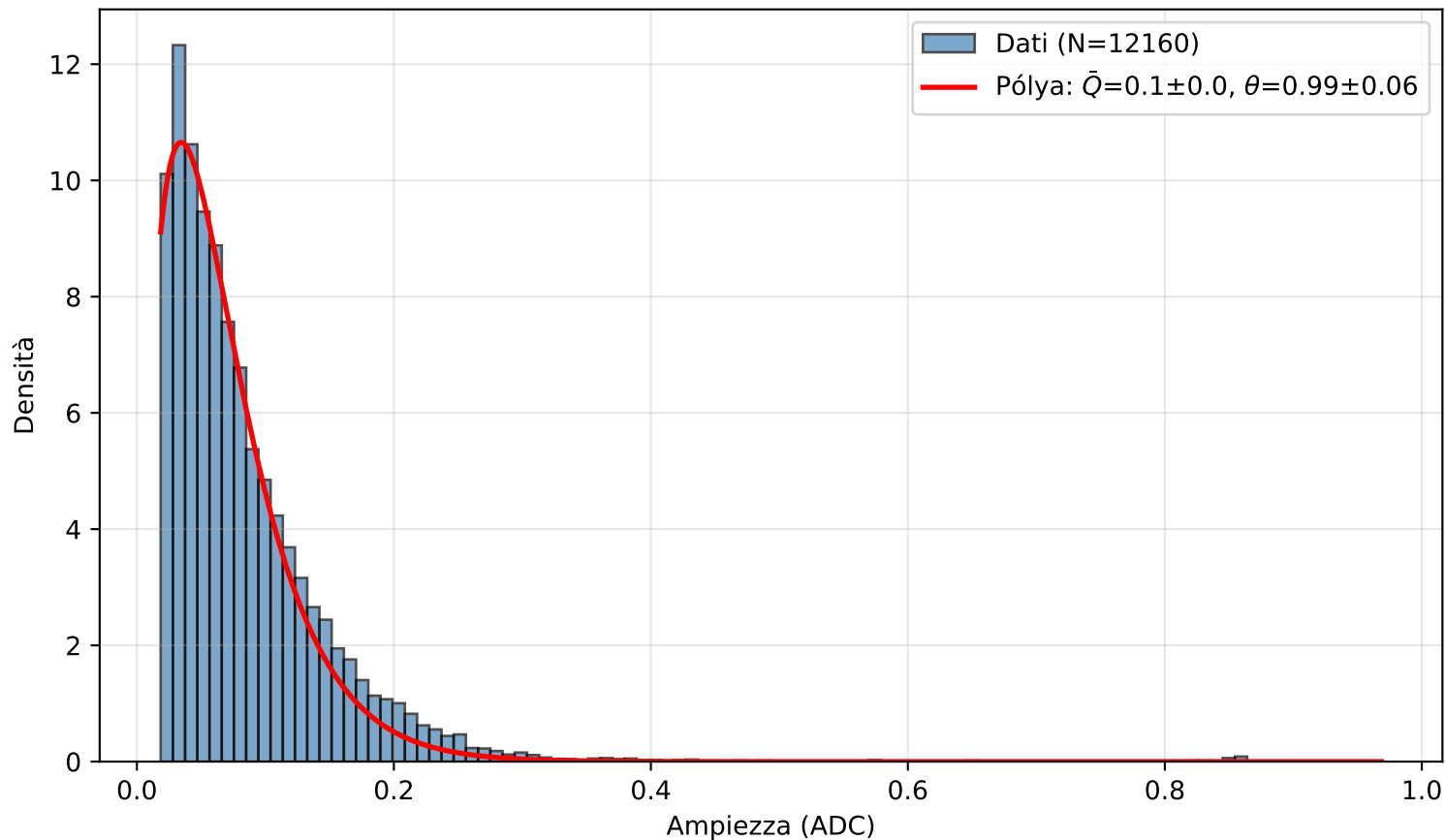
PICOSEC Detector 1 — Canale (5.0, 6.0)
