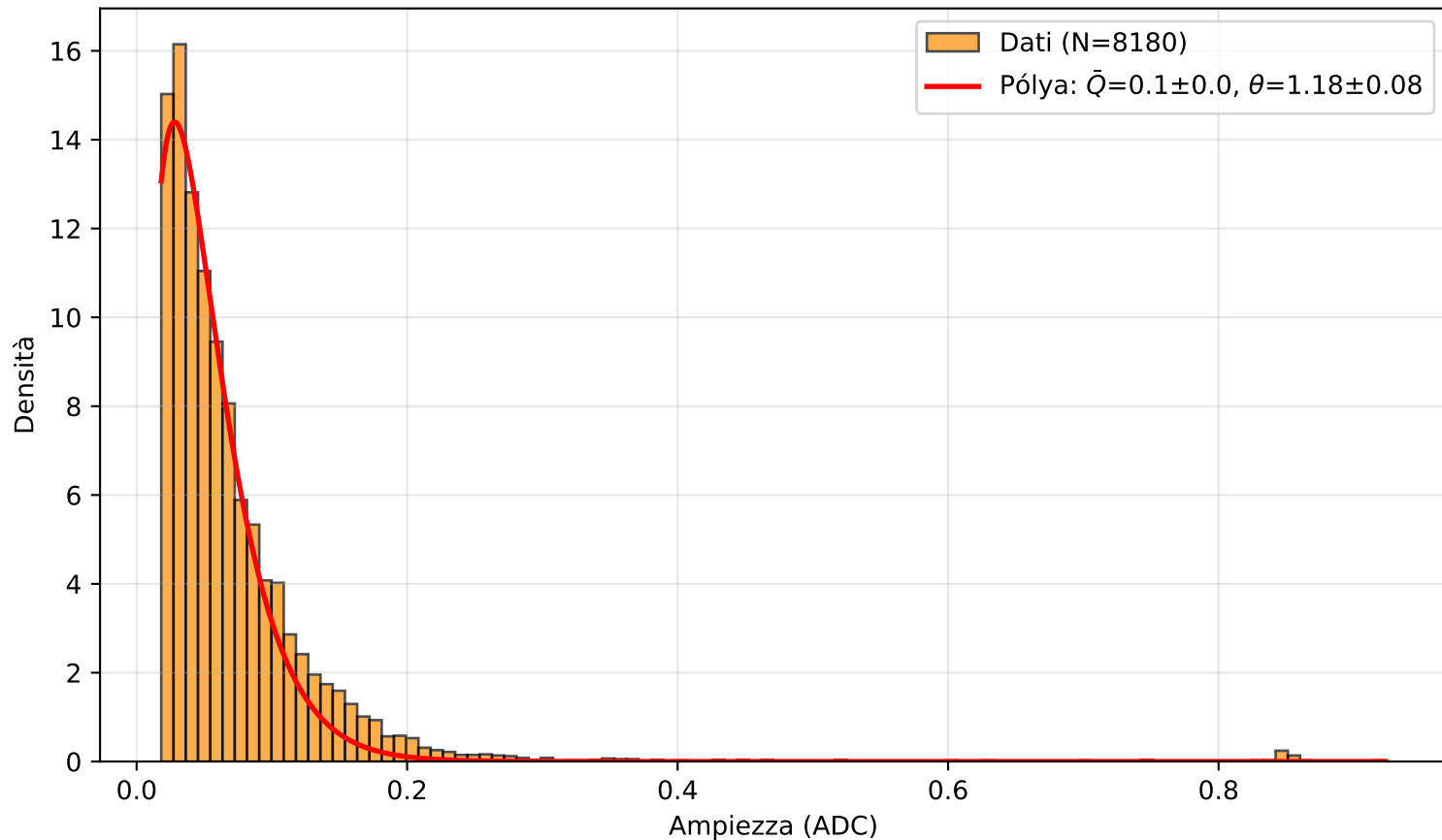
PICOSEC Detector 2 — Canale (6.0, 4.0)
