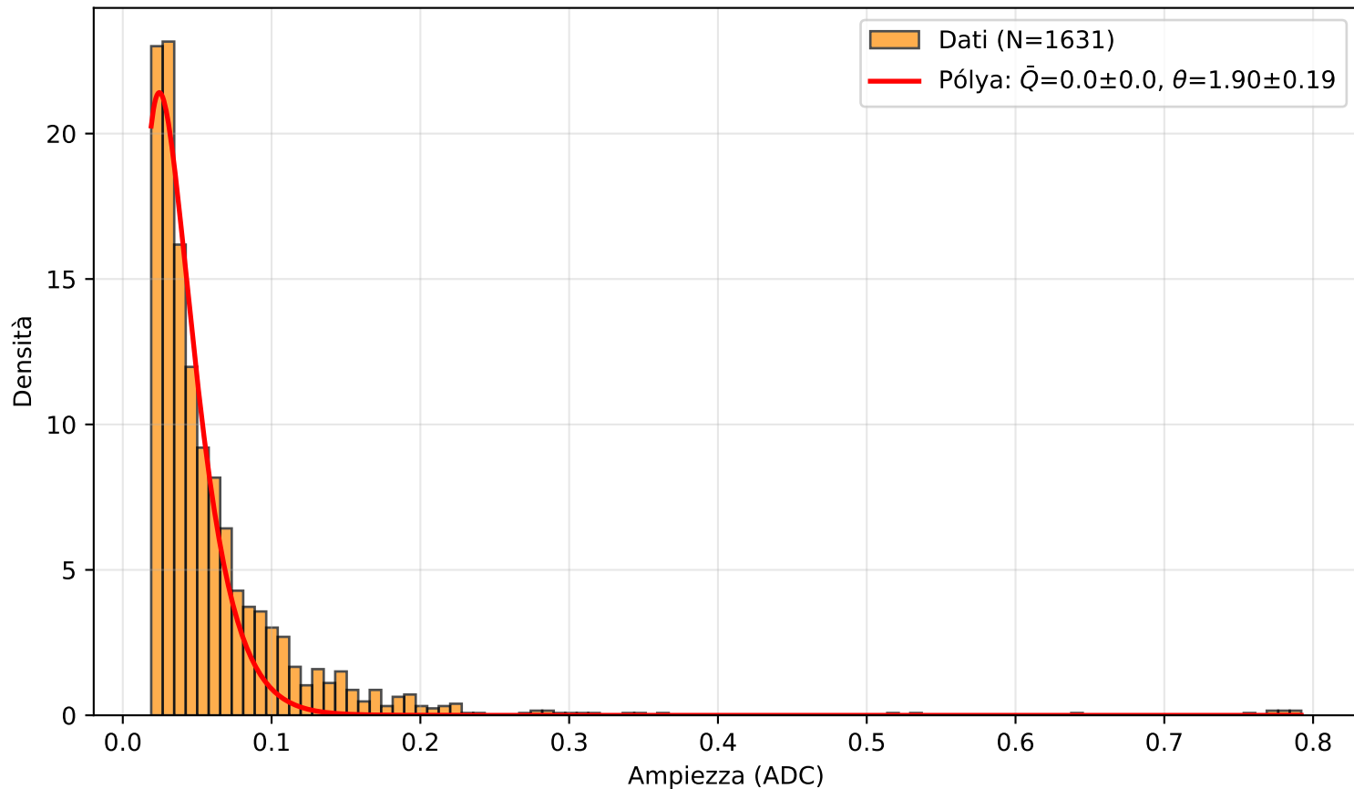
PICOSEC Detector 2 — Canale (5.0, 2.0)
