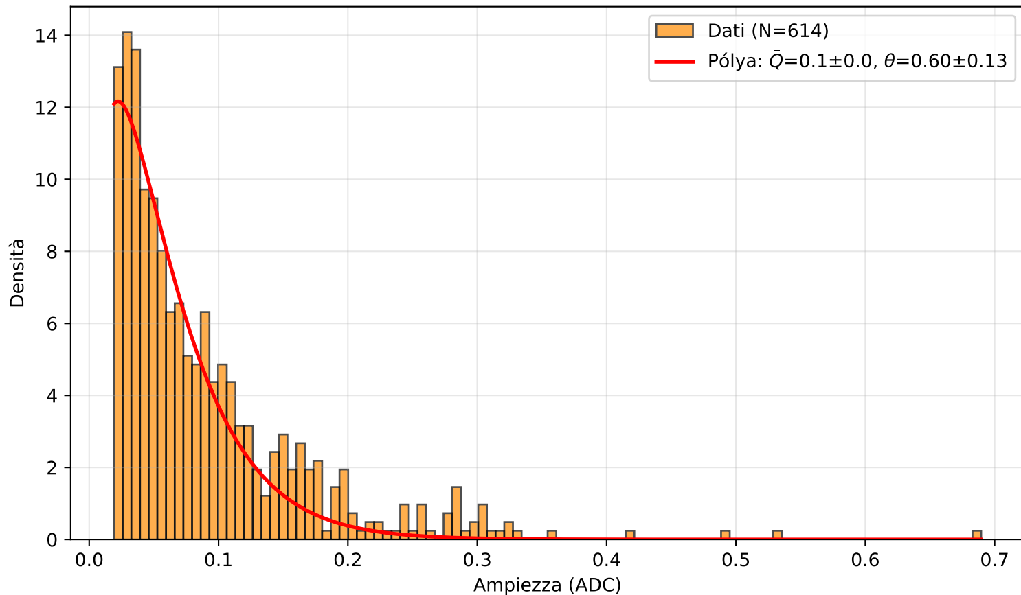
PICOSEC Detector 2 — Canale (3.0, 9.0)
