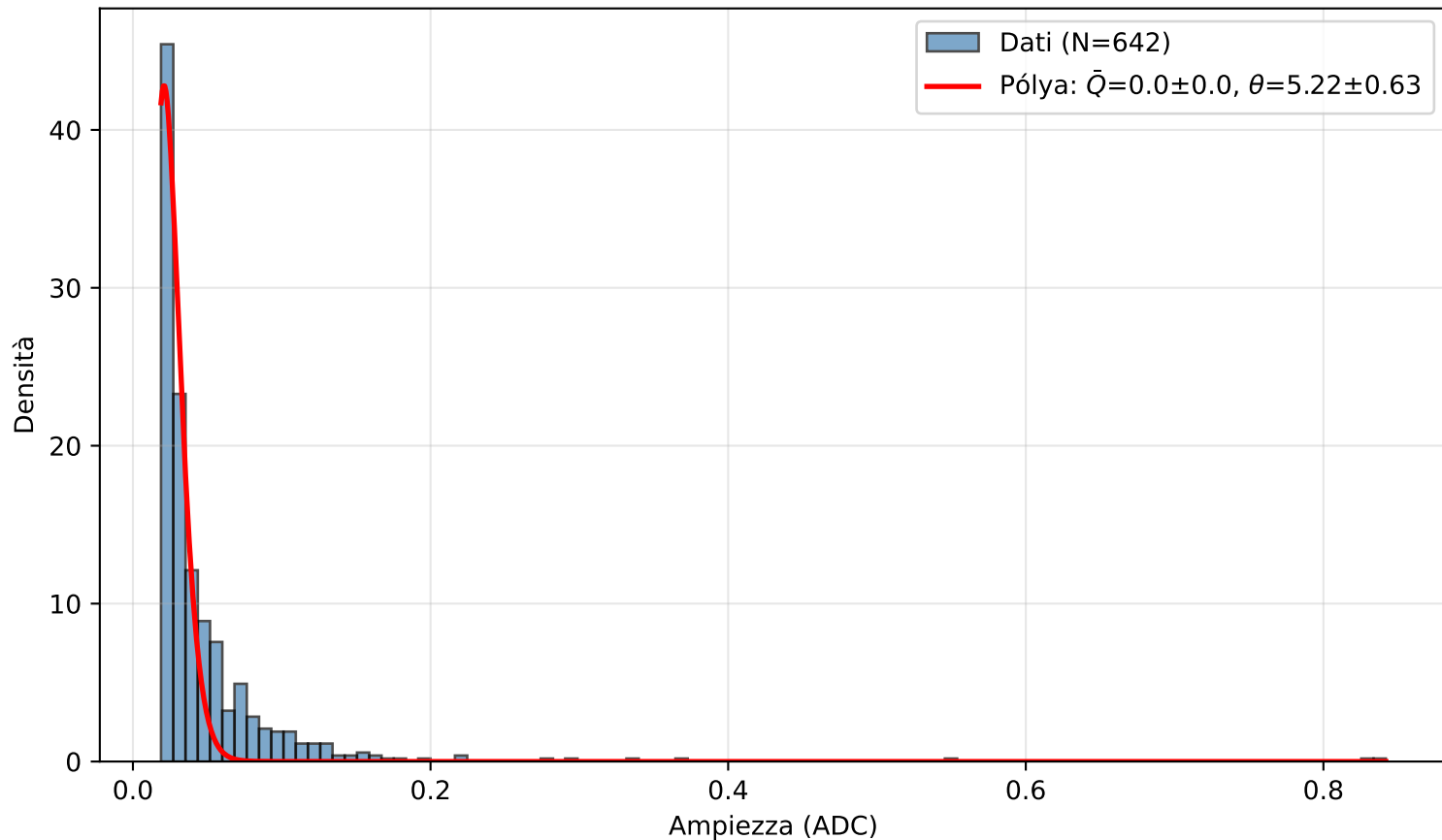
PICOSEC Detector 1 — Canale (1.0, 3.0)
