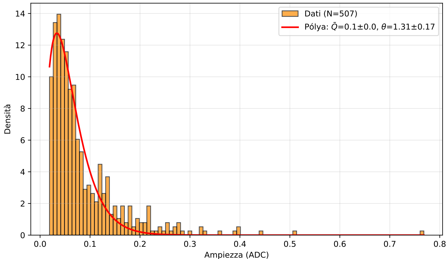
PICOSEC Detector 2 — Canale (2.0, 9.0)
