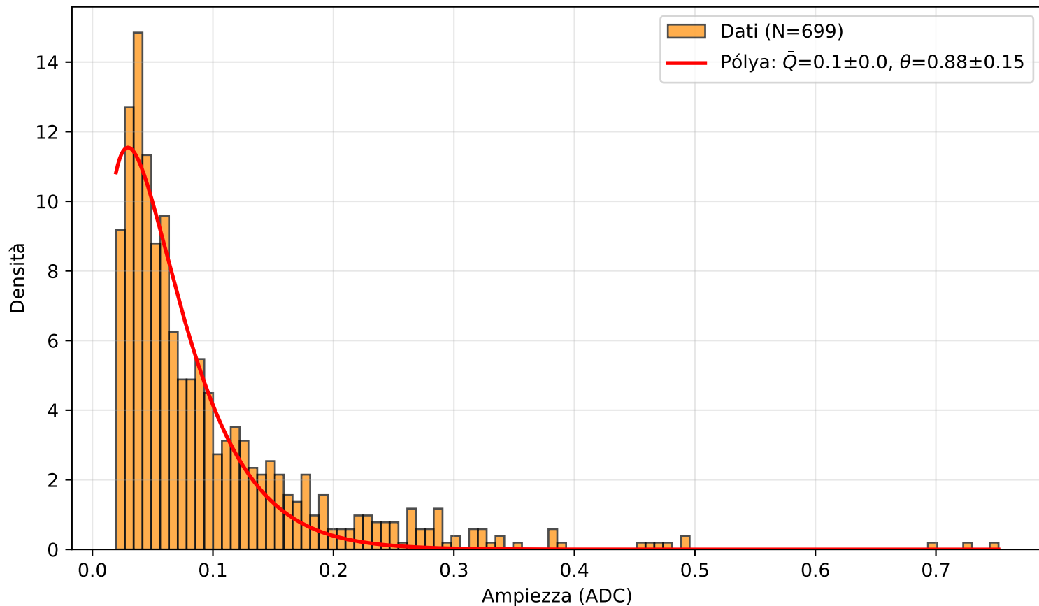
PICOSEC Detector 2 — Canale (3.0, 0.0)
