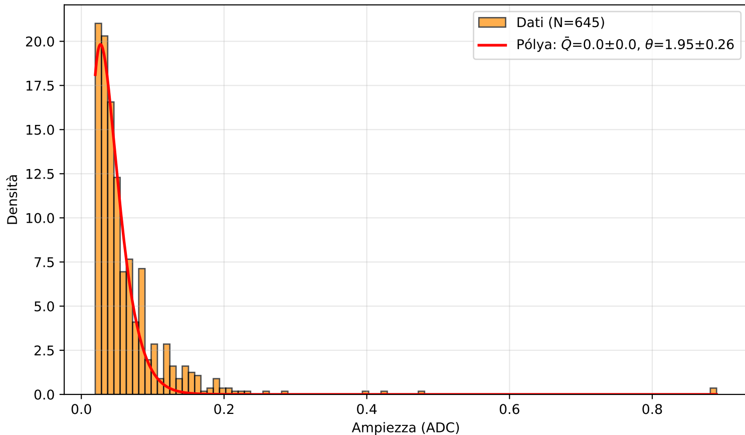
PICOSEC Detector 2 — Canale (2.0, 6.0)
