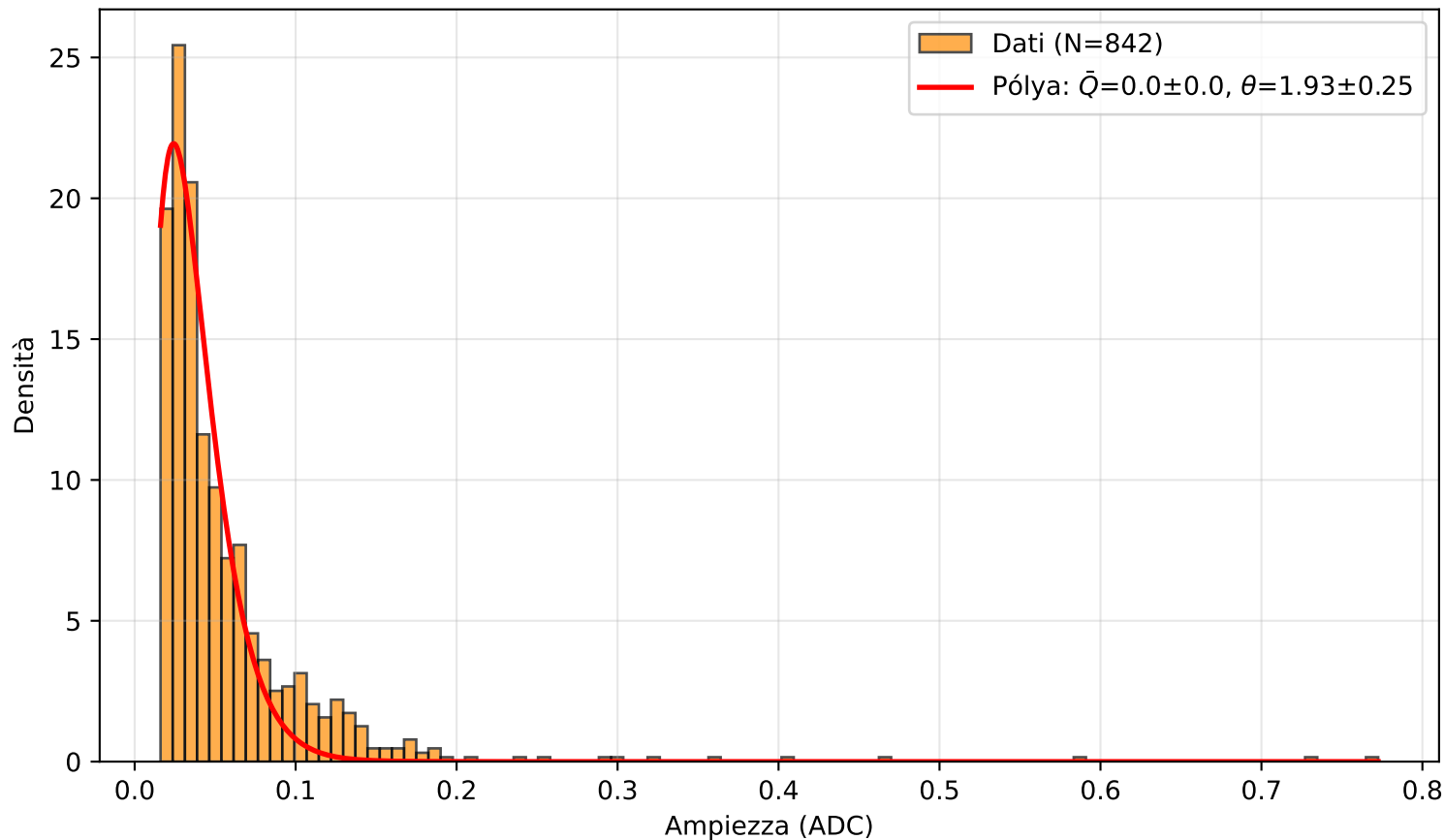
PICOSEC Detector 2 — Canale (7.0, 2.0)
