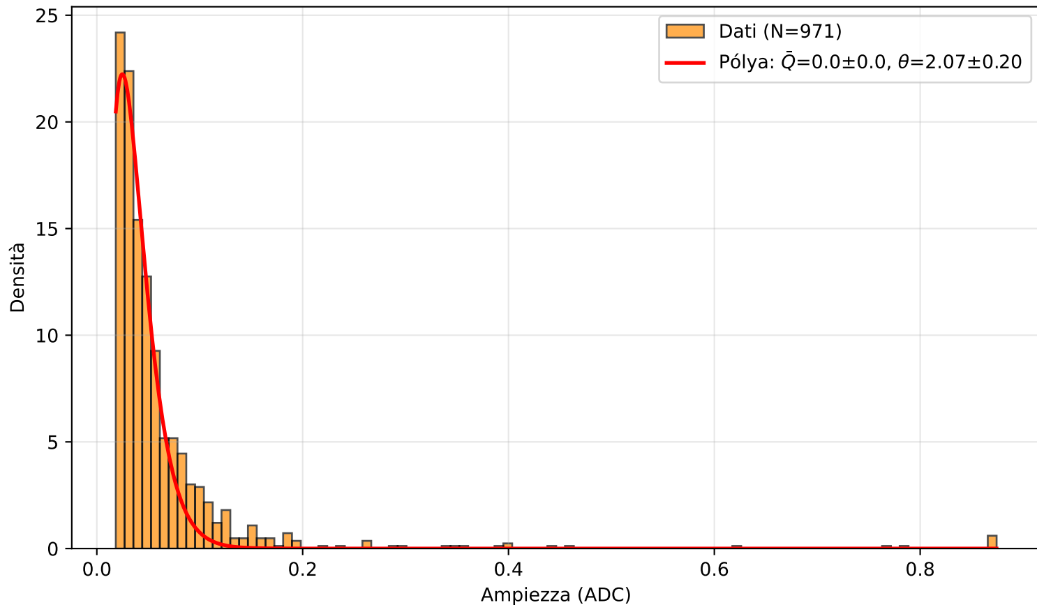
PICOSEC Detector 2 — Canale (2.0, 4.0)
