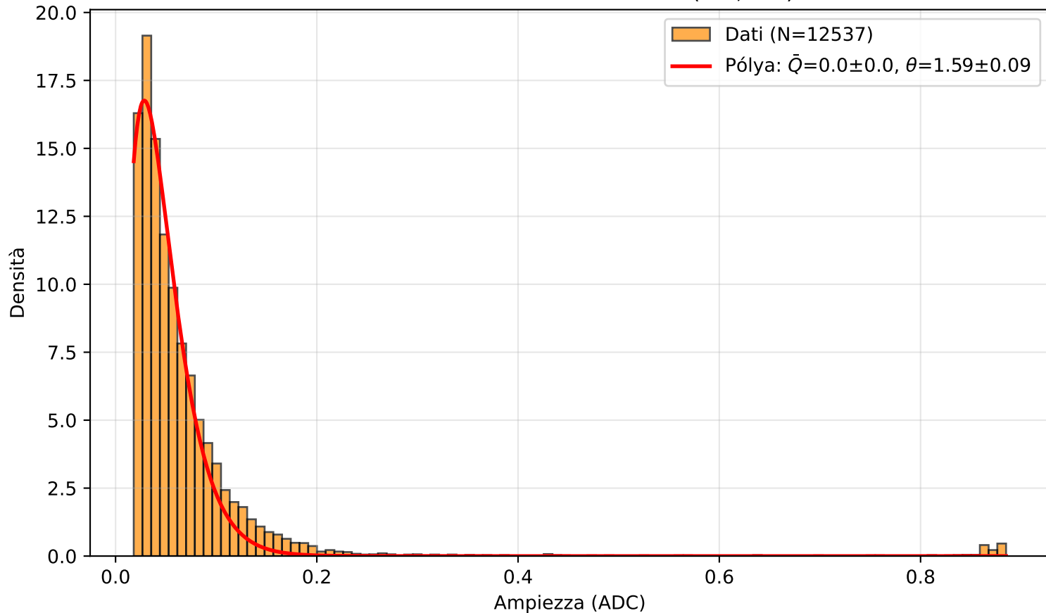
PICOSEC Detector 2 — Canale (4.0, 4.0)
