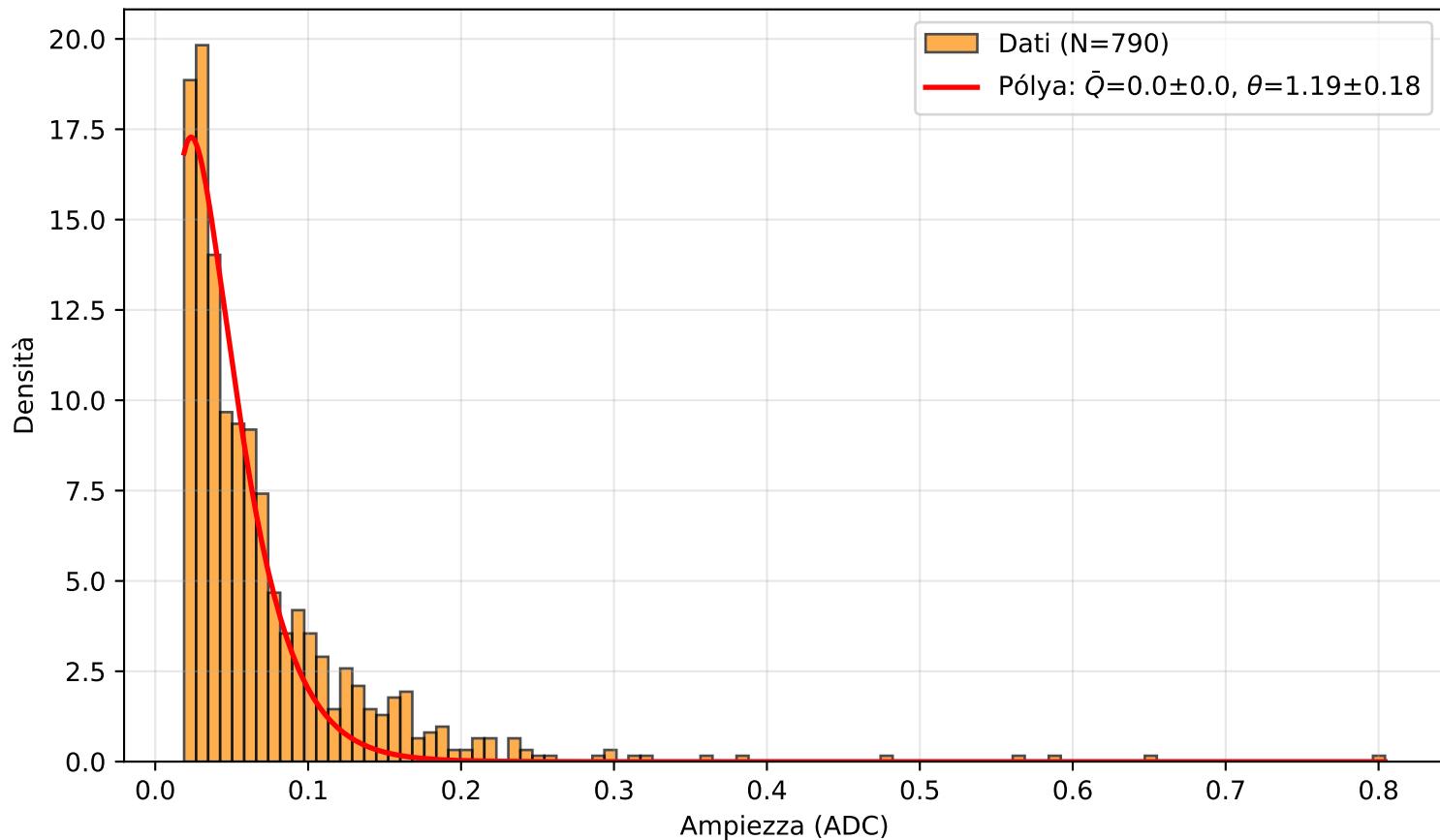
PICOSEC Detector 2 — Canale (4.0, 8.0)
