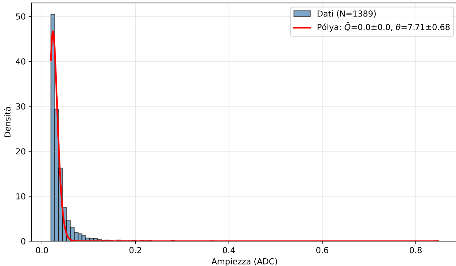
PICOSEC Detector 1 — Canale (1.0, 4.0)
