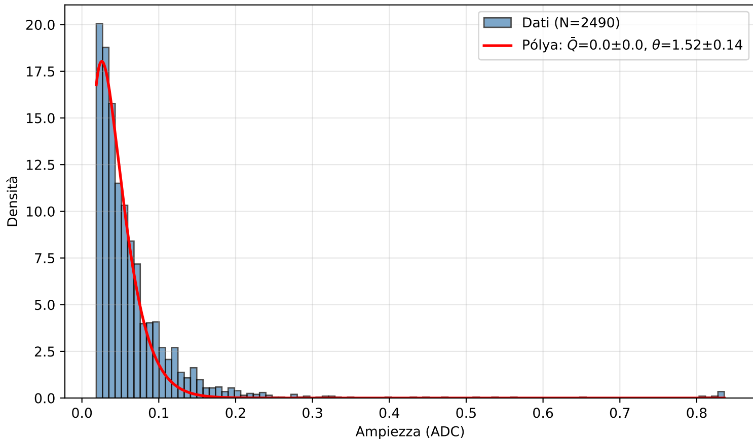
PICOSEC Detector 1 — Canale (3.0, 4.0)
