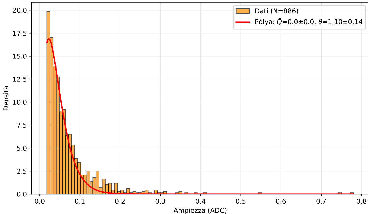
PICOSEC Detector 2 — Canale (5.0, 1.0)
