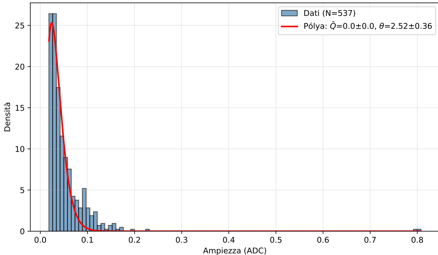
PICOSEC Detector 1 — Canale (5.0, 1.0)
