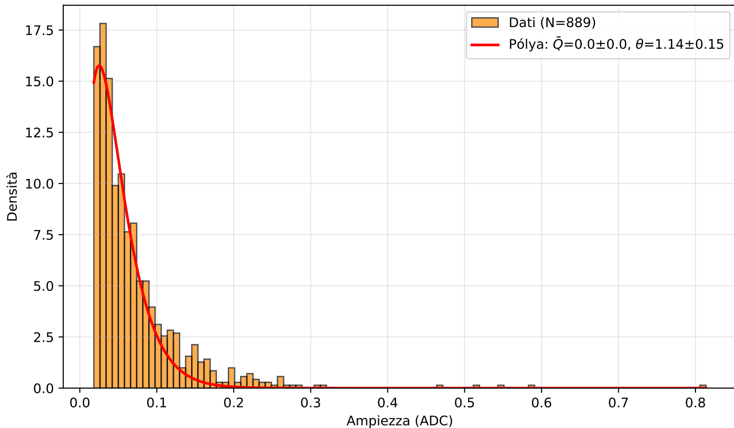
PICOSEC Detector 2 — Canale (3.0, 7.0)
