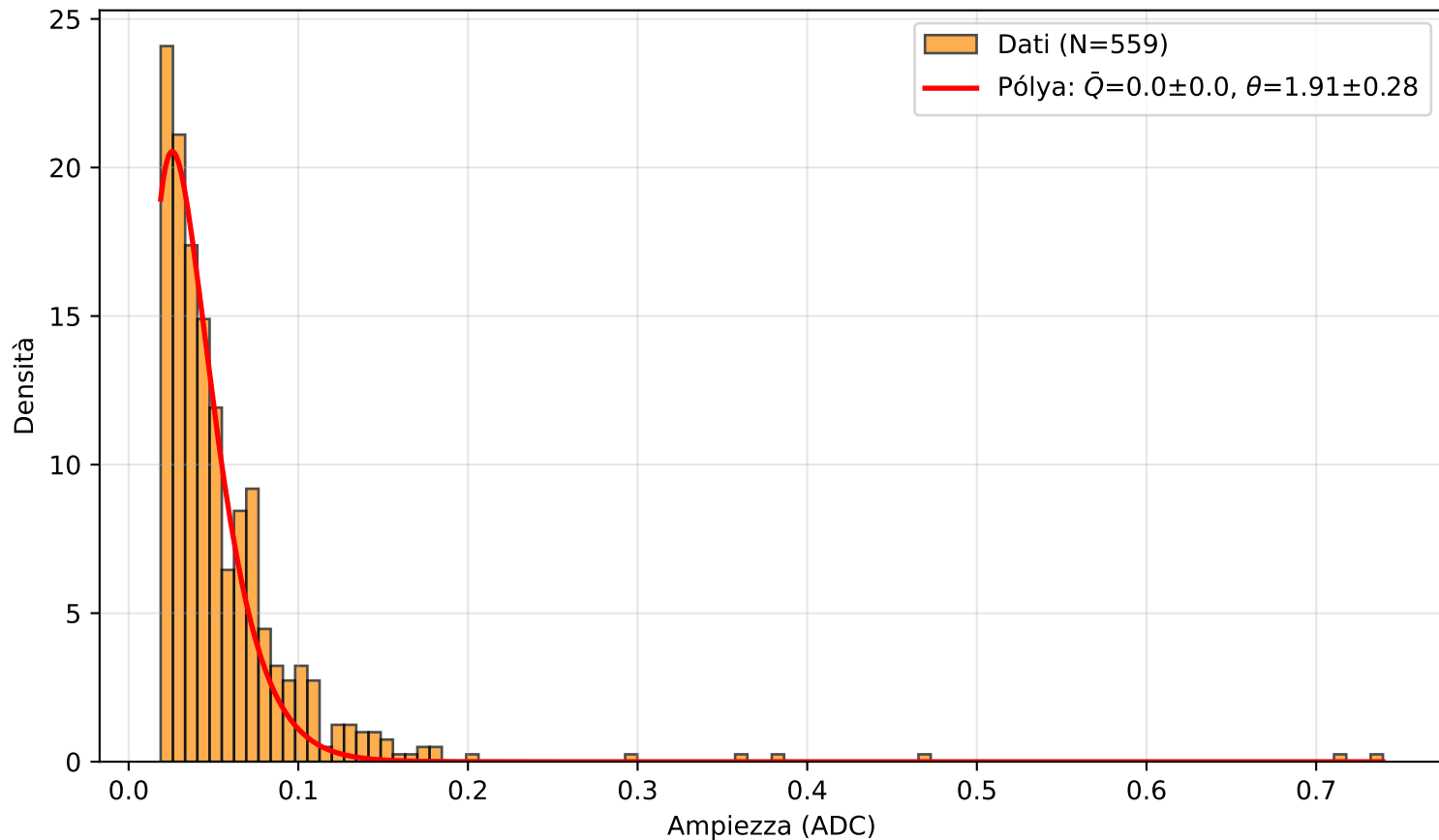
PICOSEC Detector 2 — Canale (1.0, 6.0)
