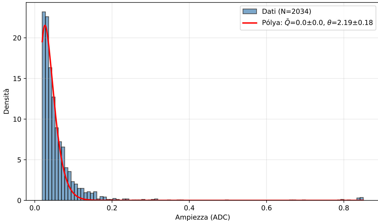
PICOSEC Detector 1 — Canale (6.0, 3.0)
