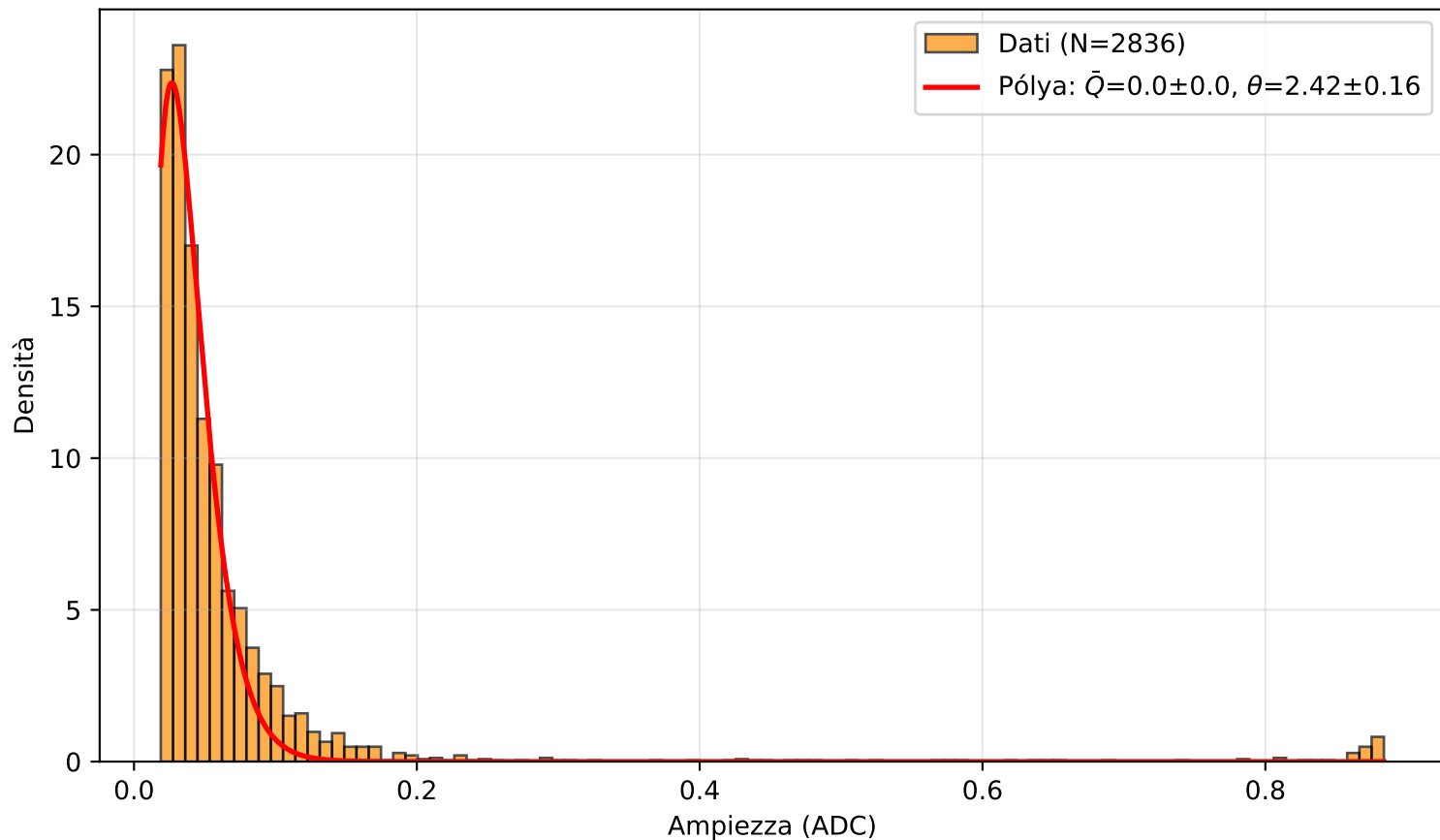
PICOSEC Detector 2 — Canale (3.0, 4.0)
