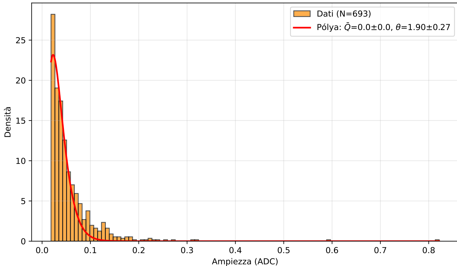
PICOSEC Detector 2 — Canale (7.0, 6.0)
