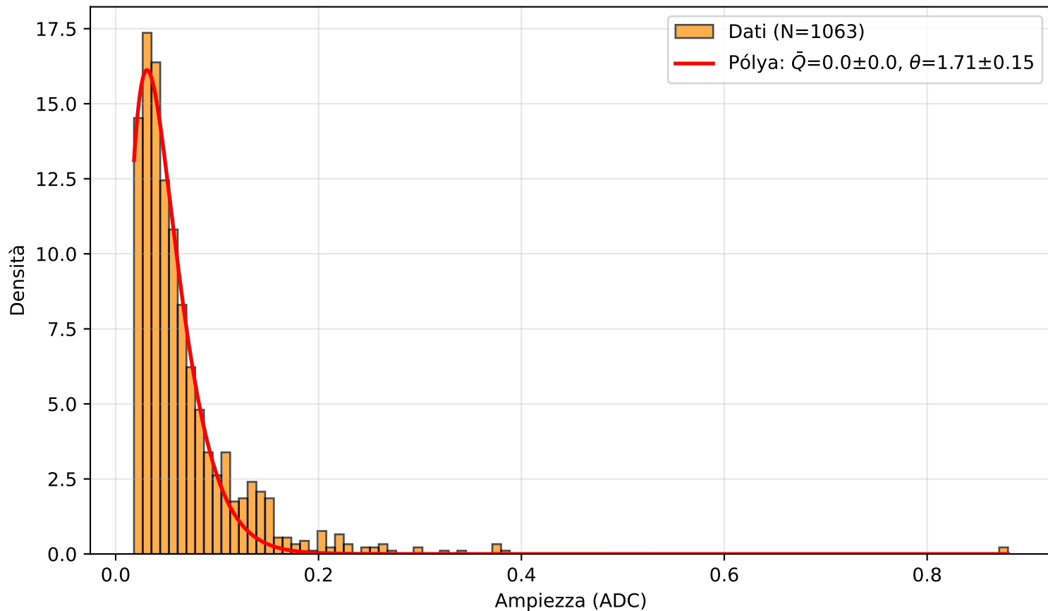
PICOSEC Detector 2 — Canale (3.0, 6.0)
