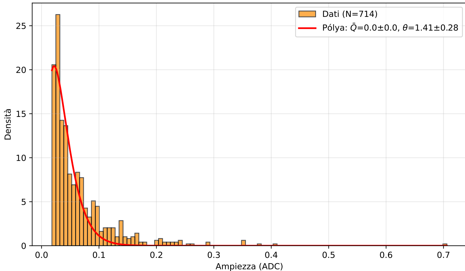
PICOSEC Detector 2 — Canale (6.0, 8.0)
