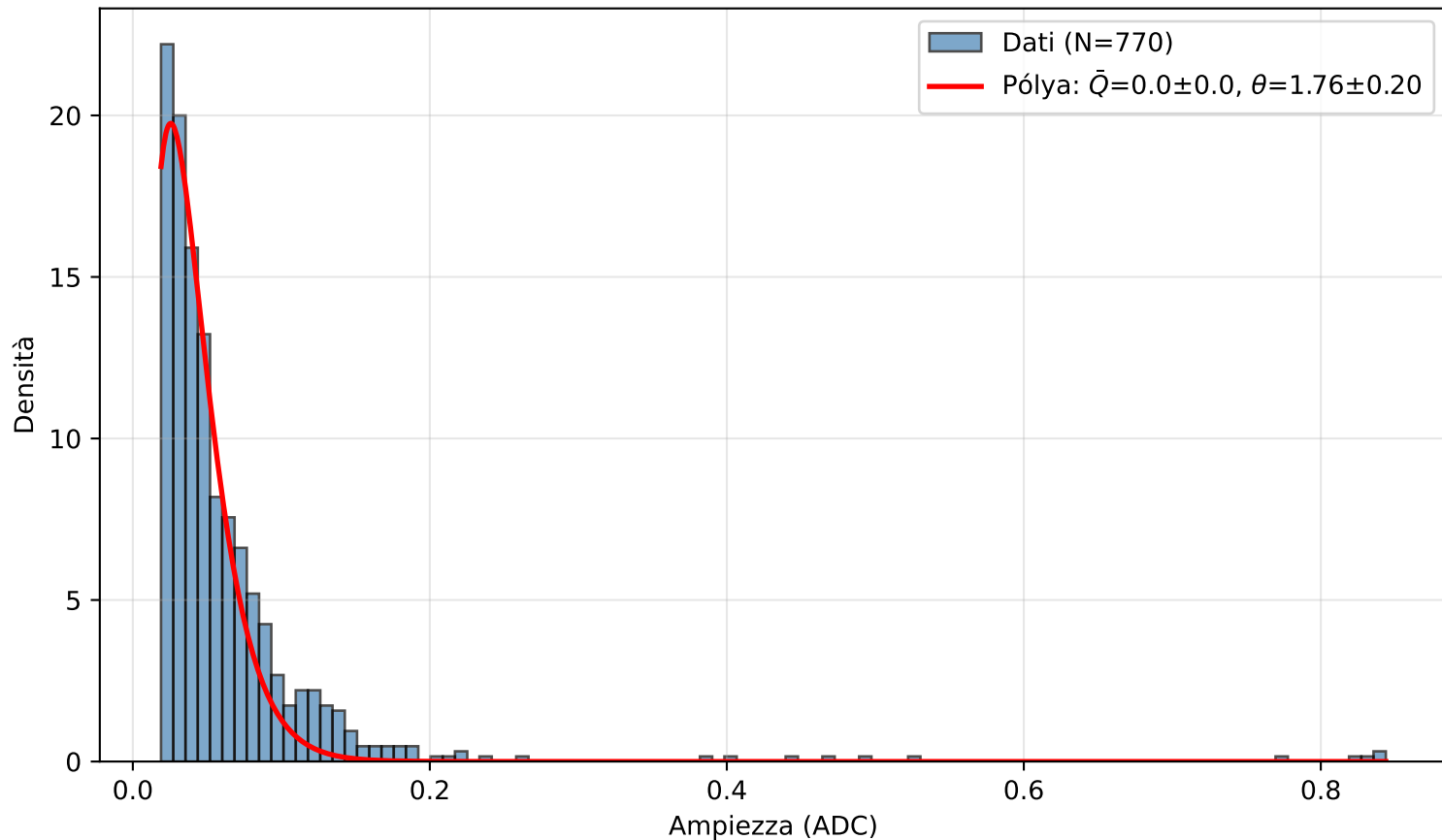
PICOSEC Detector 1 — Canale (2.0, 2.0)
