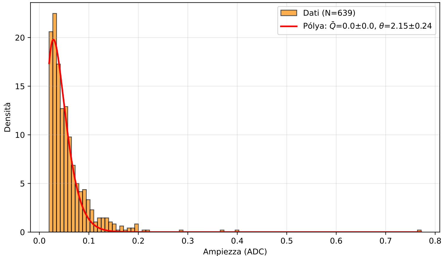
PICOSEC Detector 2 — Canale (2.0, 1.0)
