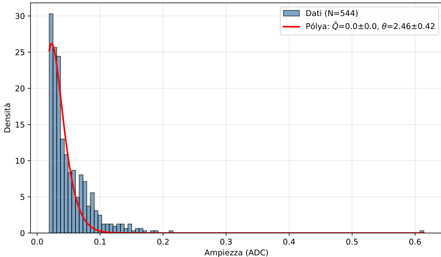
PICOSEC Detector 1 — Canale (6.0, 8.0)
