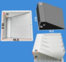
路肩模具 49.8*49.8*26cm 49.8x49.8x26 路肩
