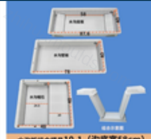
水沟板组合模具10-1 (沟底宽58cm)
