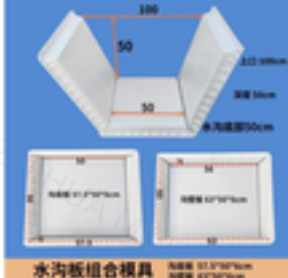
水沟板组合模具 上口100 下口50 深度50 水沟板
