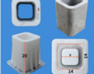
方孔空心砖 14*14*20cm 14x14x20cm 方孔
