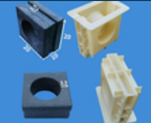
空心砖 圆孔三合一 20*20*10cm 20x20x10 ABS圆孔三合一
