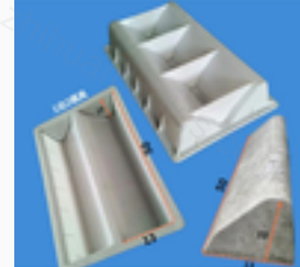
坡型排水路沿石 50*13*10cm 50*13*10 排水石 (1出2)
