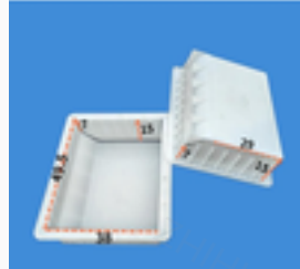
坡型路沿石 49.5*38*15cm 49.5x38x15 坡型路沿石
