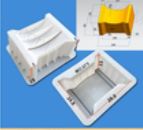
凹面缺口盖板 28.8*24.8*15cm 28.8x24.8x15 凹面缺口盖板
