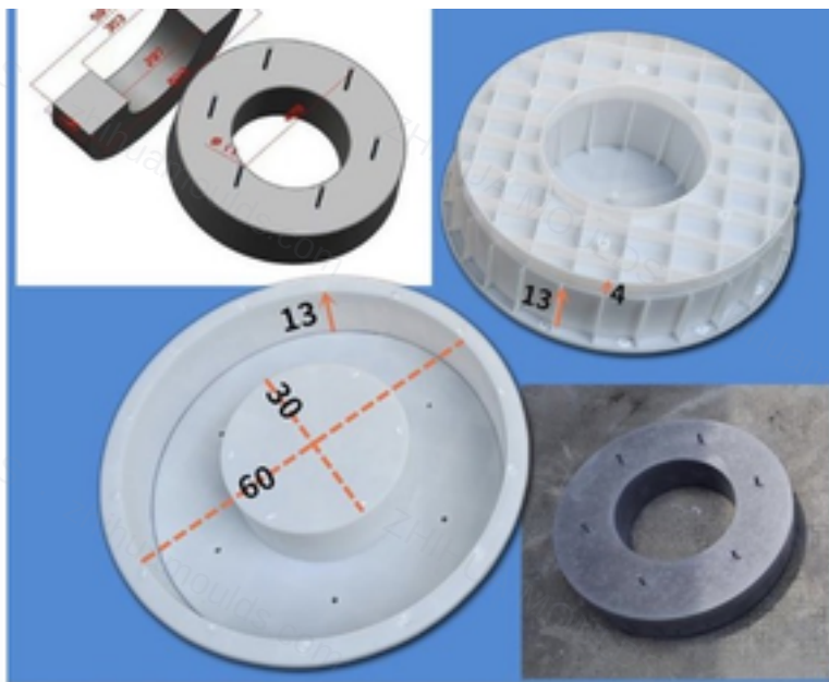
圓形水泥基座模具 直径60 孔径30 厚度13cm
