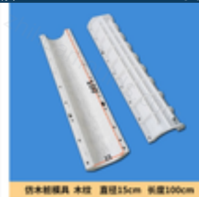
仿木桩模具 木纹 直径15cm 长度100cm 直径15 长度100 木纹仿木桩
