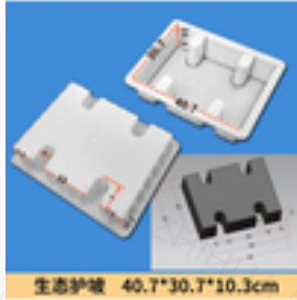
生态护坡 40.7*30.7*10.3cm 40.7x30.7x10.3 生态护坡
