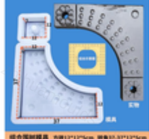
组合围树模具 方槽12*12*5cm 圆角12*12*5cm 组合式围树 12*12*5 37*37*12*
