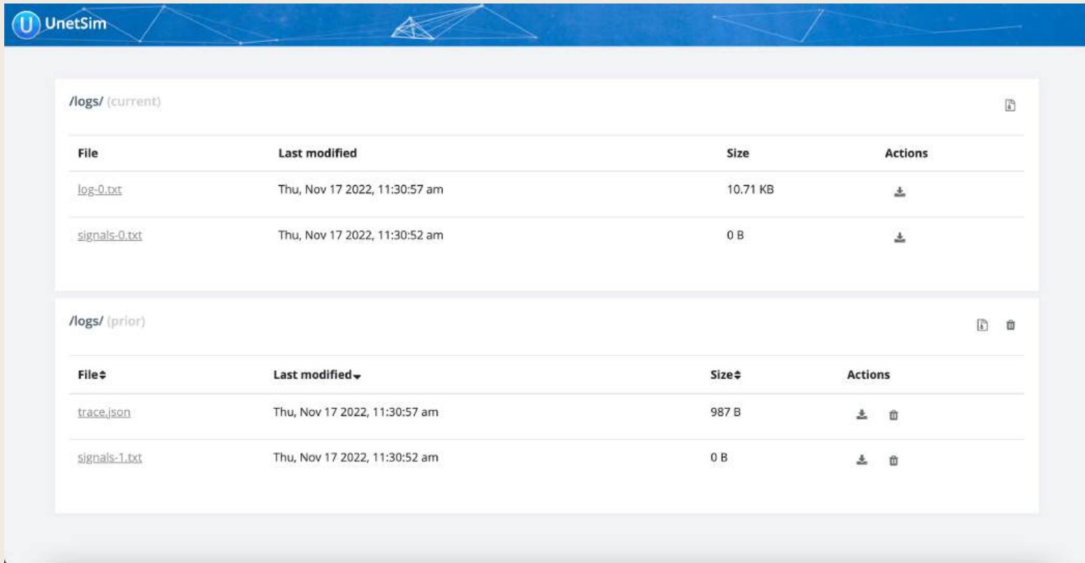
UnetSim - Logs
