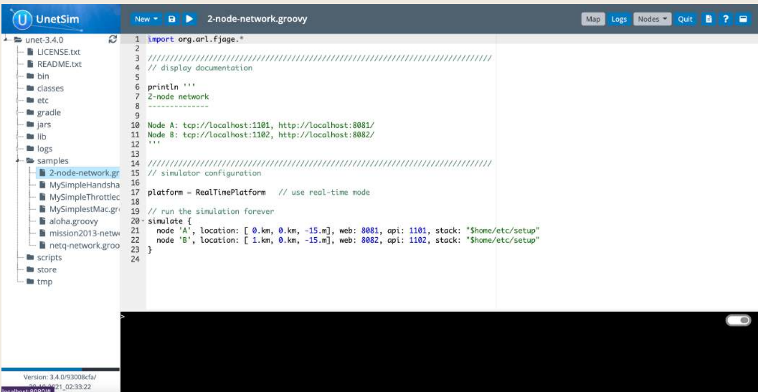
UnetSim - Editor
