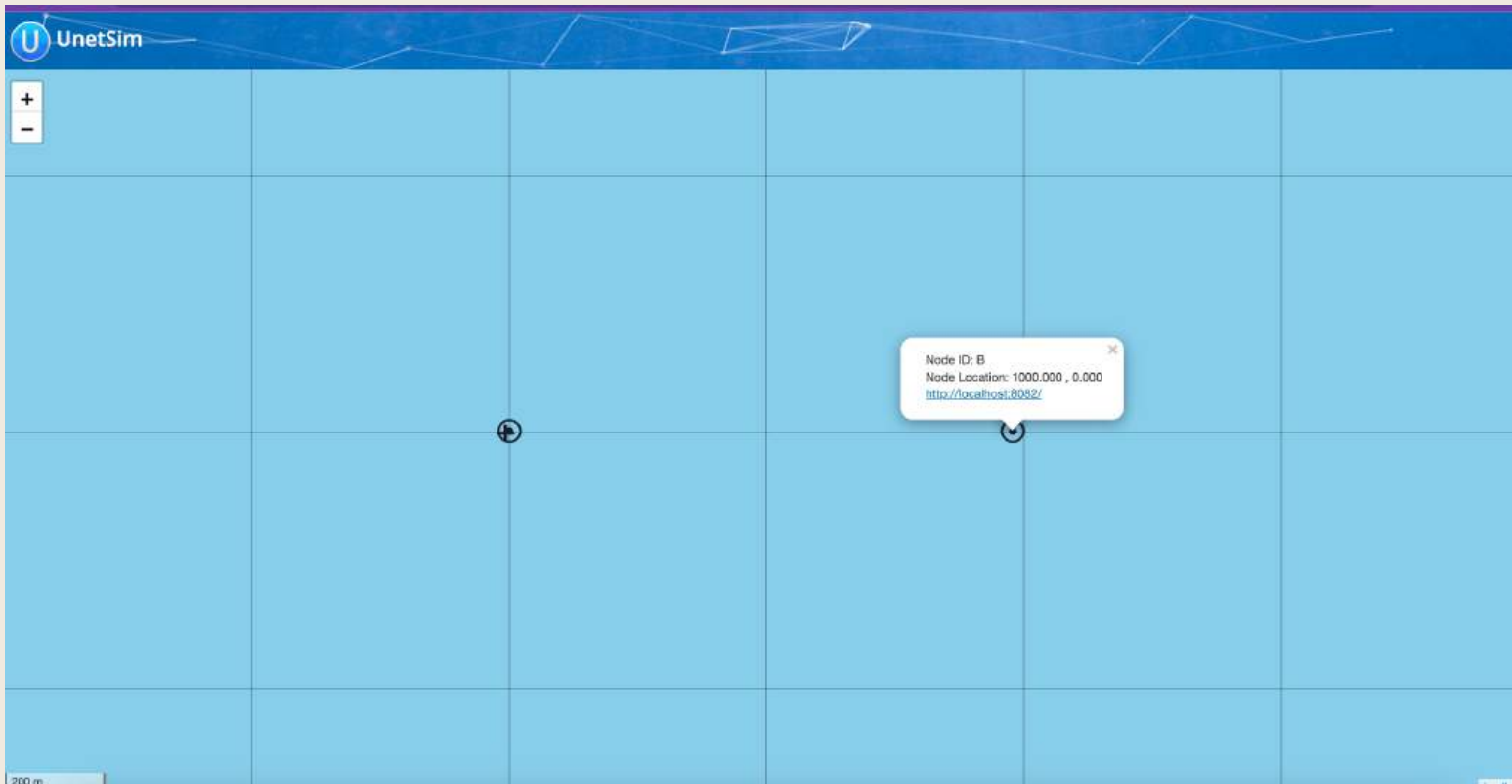
UnetSim - Map
