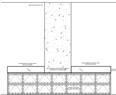
Maatwerk 8 (adeblok VA) 1:20
