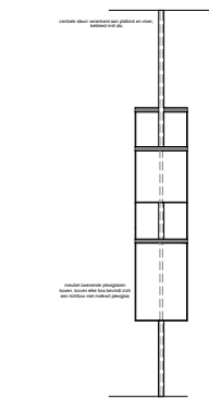
Maatwerk 10 (rek links achterwand ZA) 1:20
