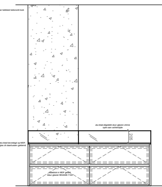
Maatwerk 7 (adeblok VA) 1:20
