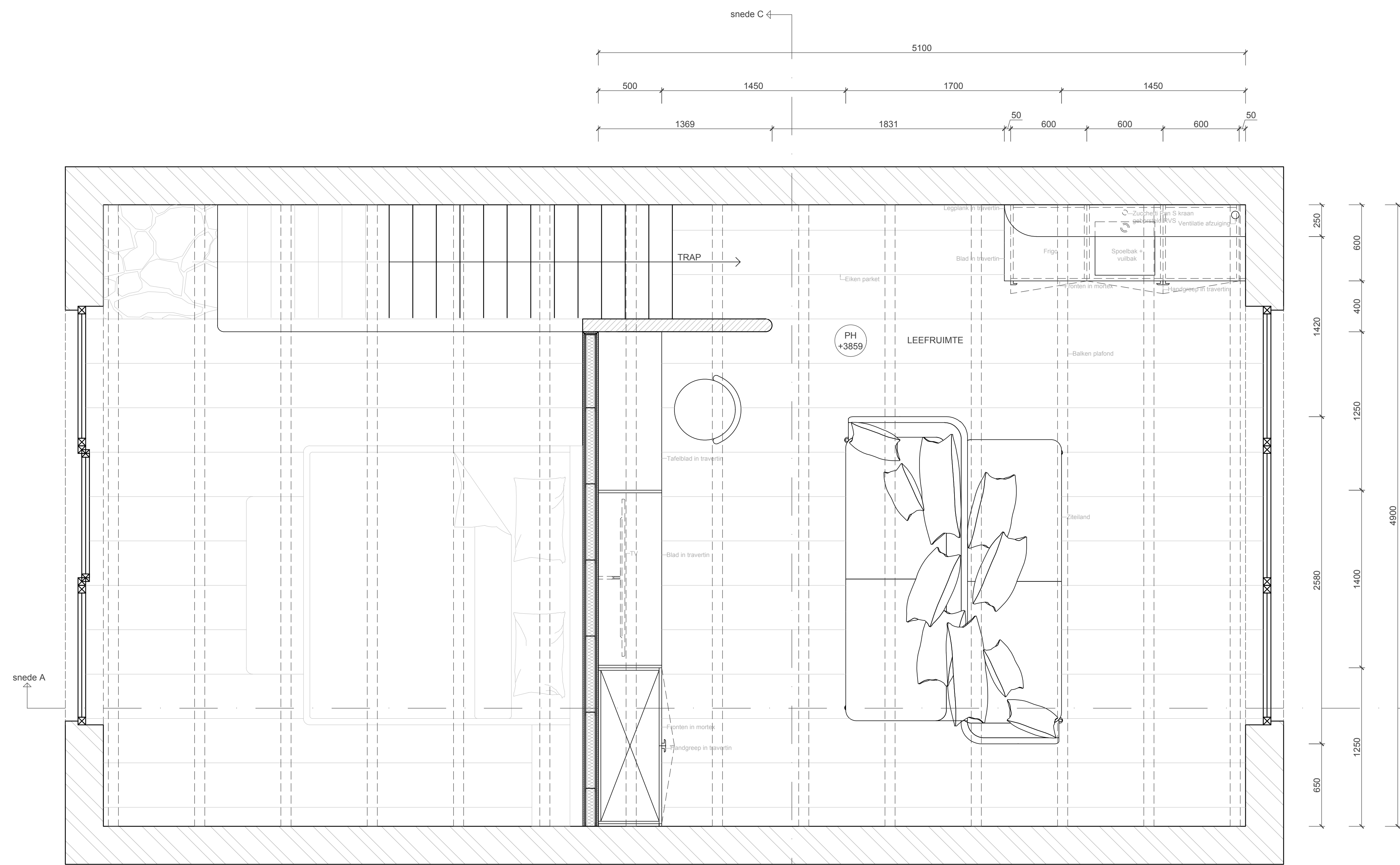
PLATTEGROND EERSTE VERDIEP 1:20
