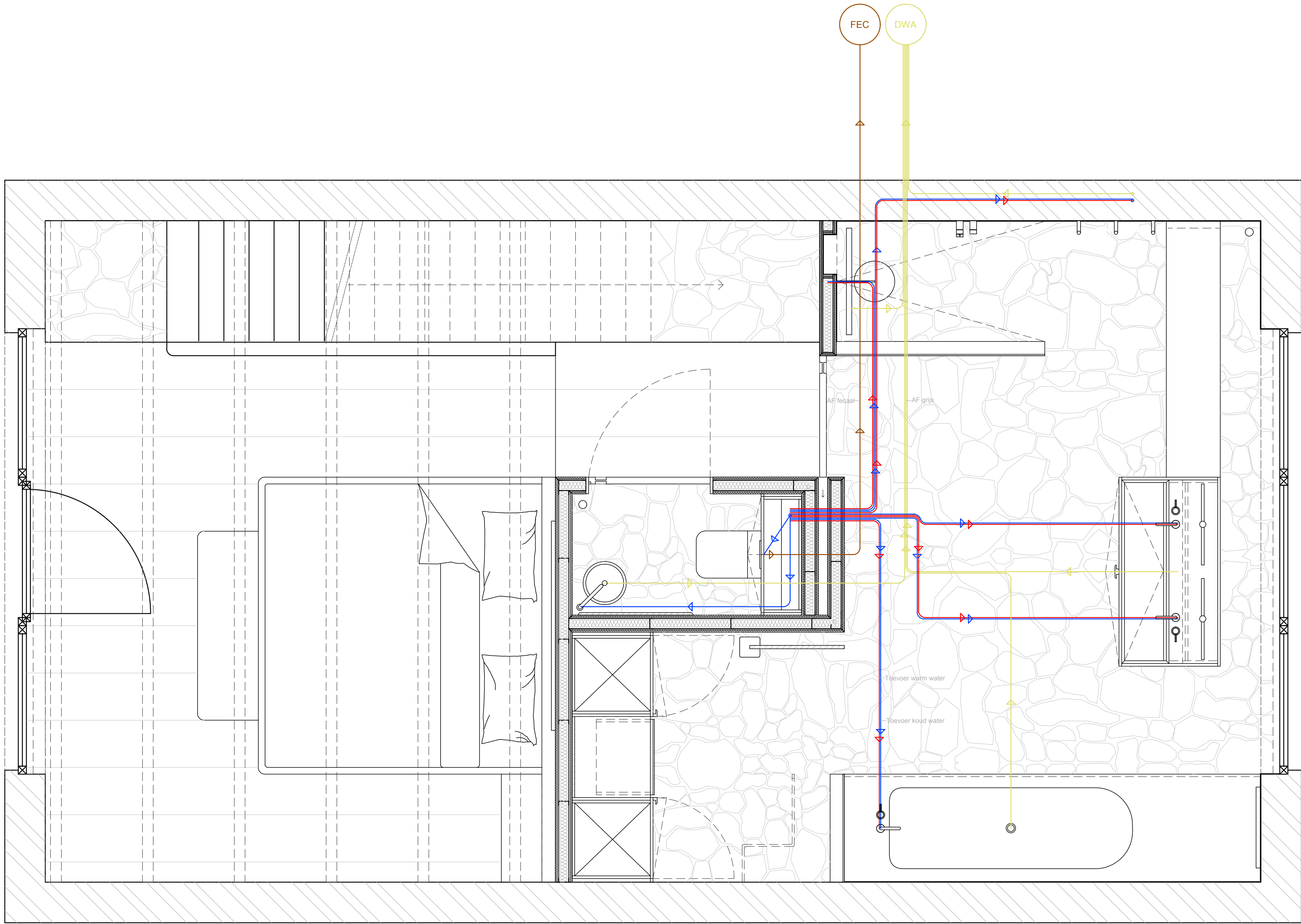
TECHNISCH PLAN GELUKVLOERS (sanitair) 1:20
