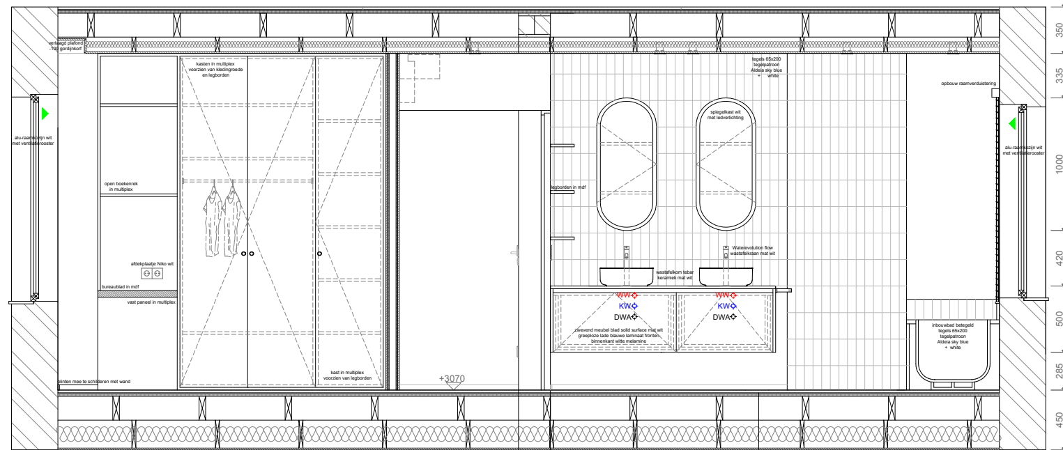
SNEDE G 1:20 (badkamer & slaapkamer 1)
