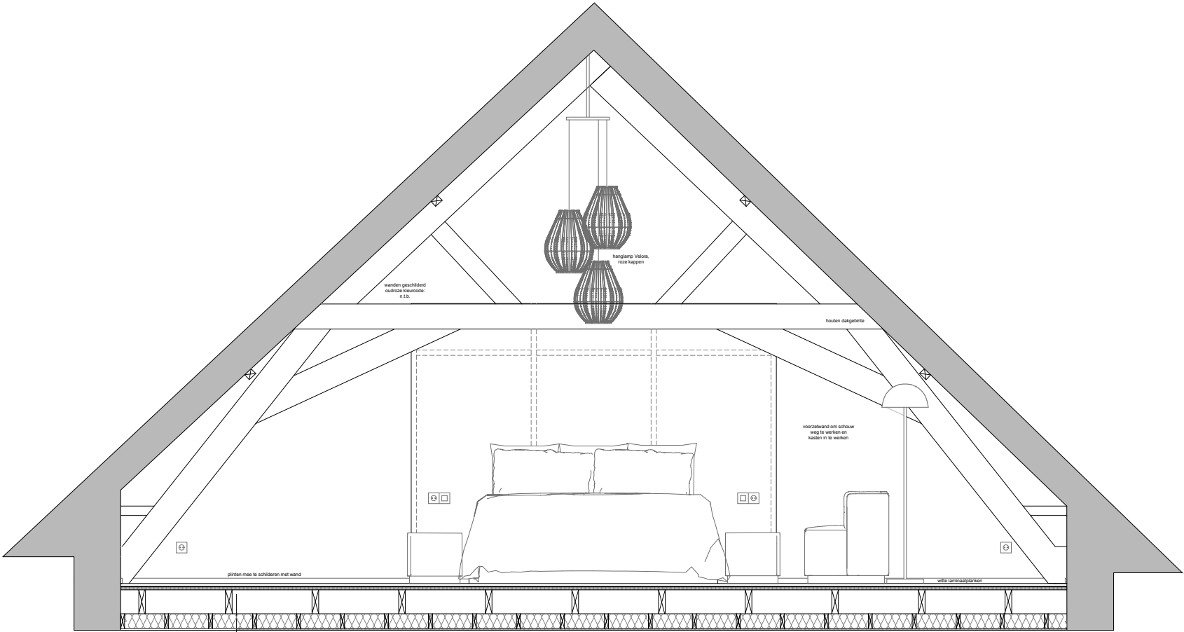
SNEDE K 1:20 (slaapkamer 3)
