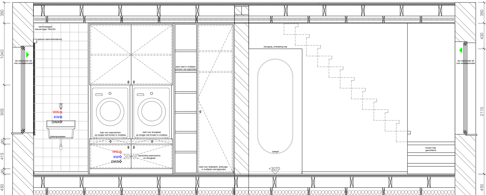
SNEDE I 1:20 (slaapkamer 2, badkamer & wasplaats)
