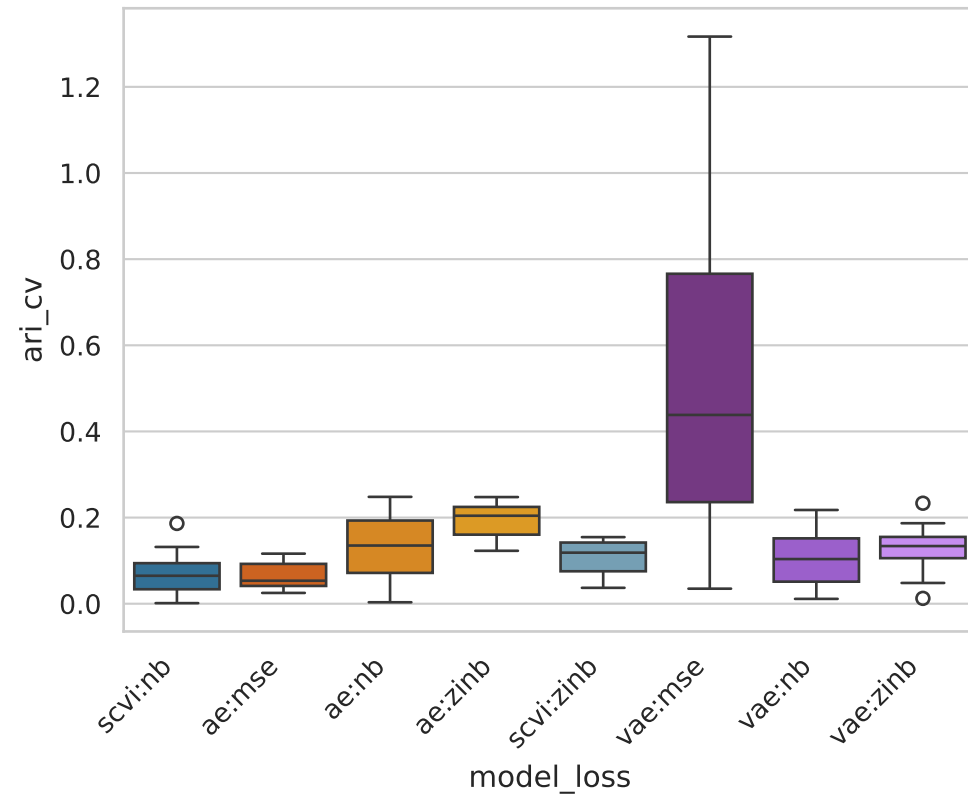
ARI CV
