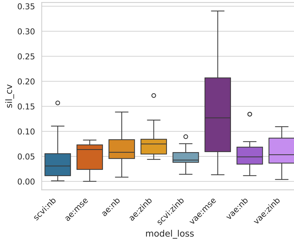
Silhouette CV
