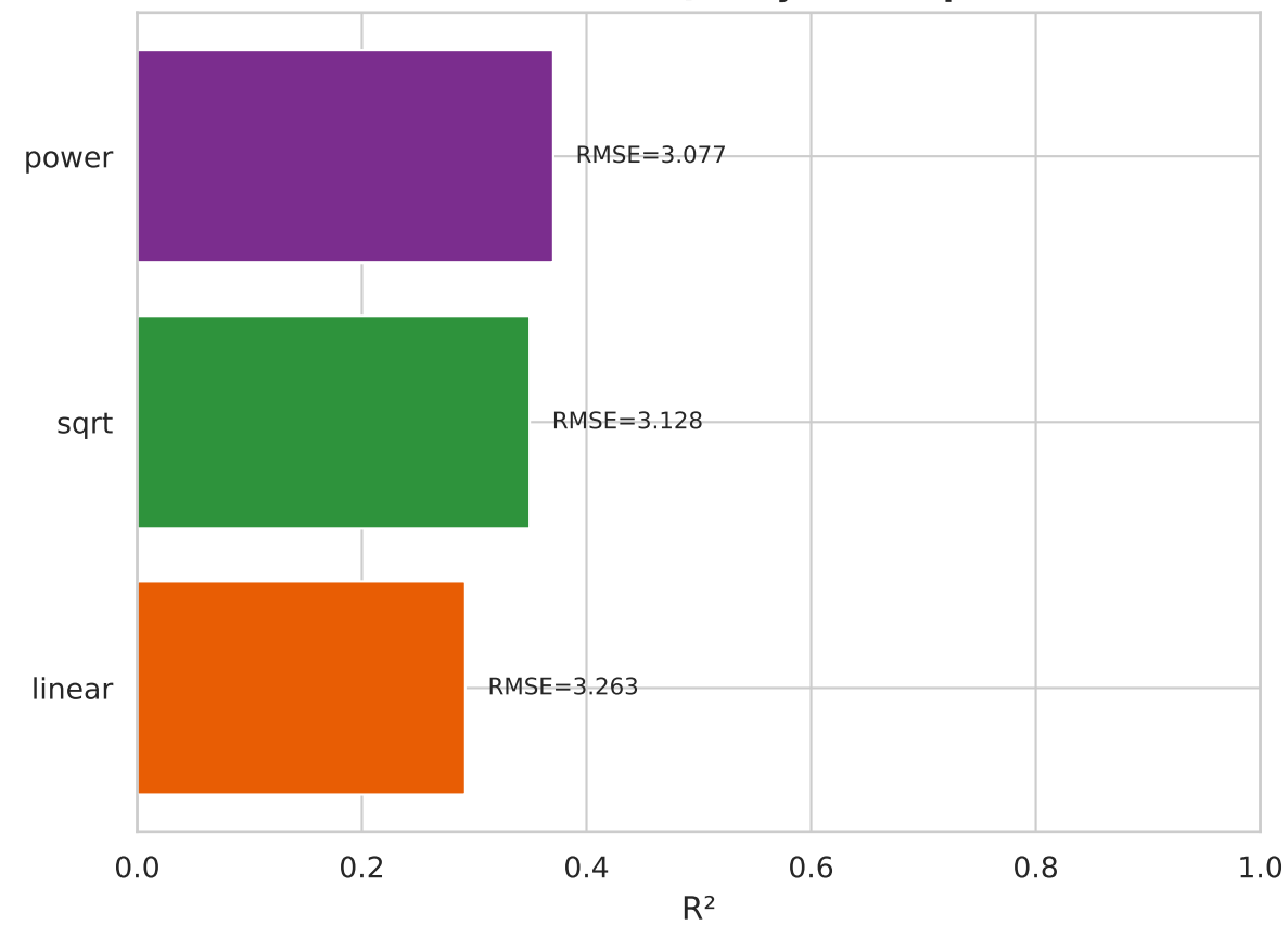
(D) Formula Fit Quality (in-sample)
