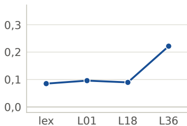
token previsto
