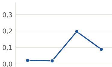
sentença
