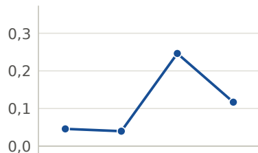
próximo token
