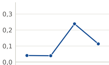
token previsto
