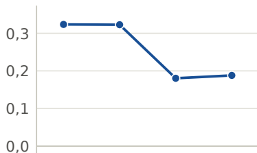
parágrafo
