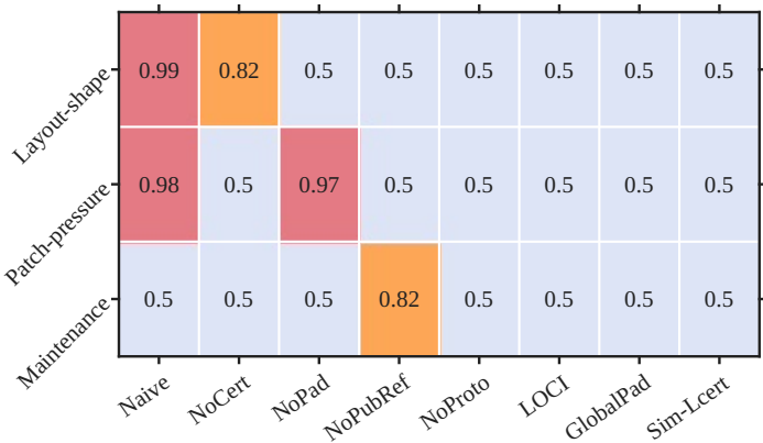
(a) TraceProbe attack AUC
