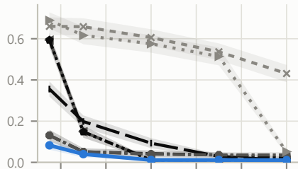
Gamma-ray survey (Fermi-LAT)
