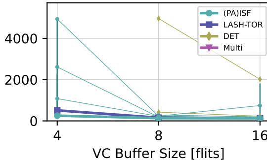
NoC (Mesh)
