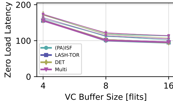
NoC (Mesh)
