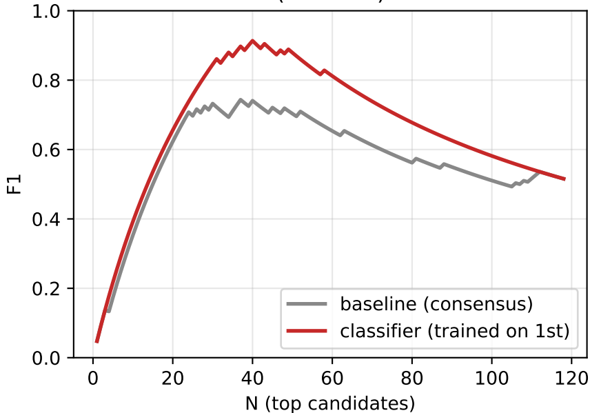
2nd half (held-out): F1 vs N
