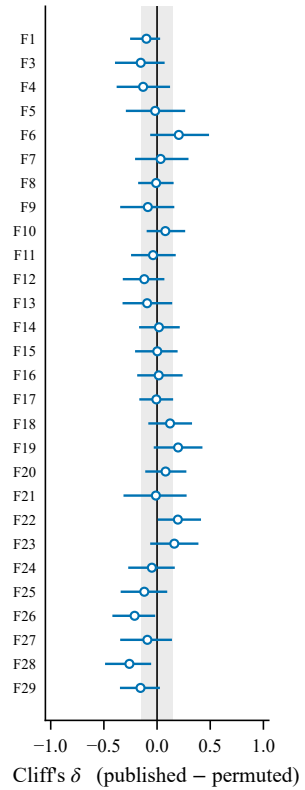
CEC2017 D=30 , 300 000 evals
