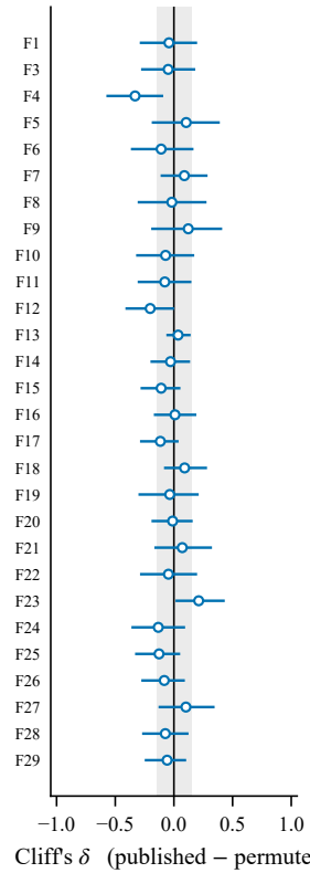
CEC2017 D=50 , 500 000 evals
