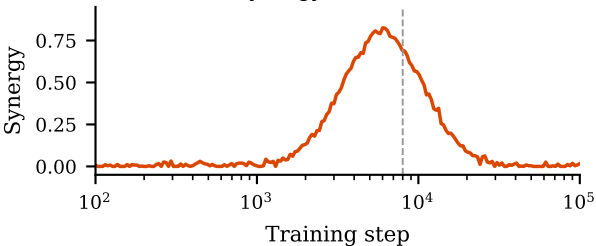
(c) Synergy (Clauw et al.)
