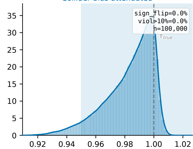
(d) Collider
