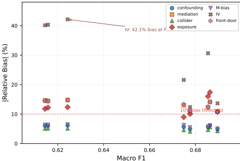
HumAID (K=10): Topology Determines Bias, Not F1
