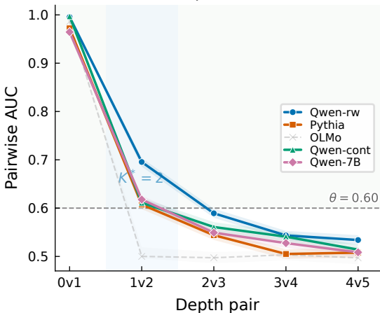
(a) Pairwise AUC profile
