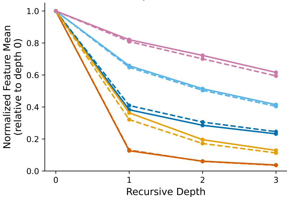
Pythia-1.4B
