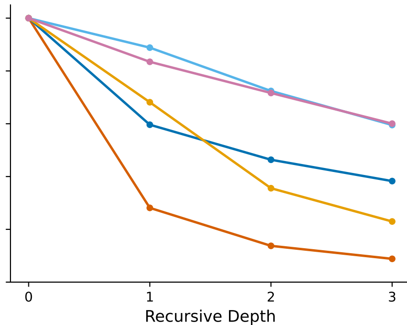
OLMo-1B
