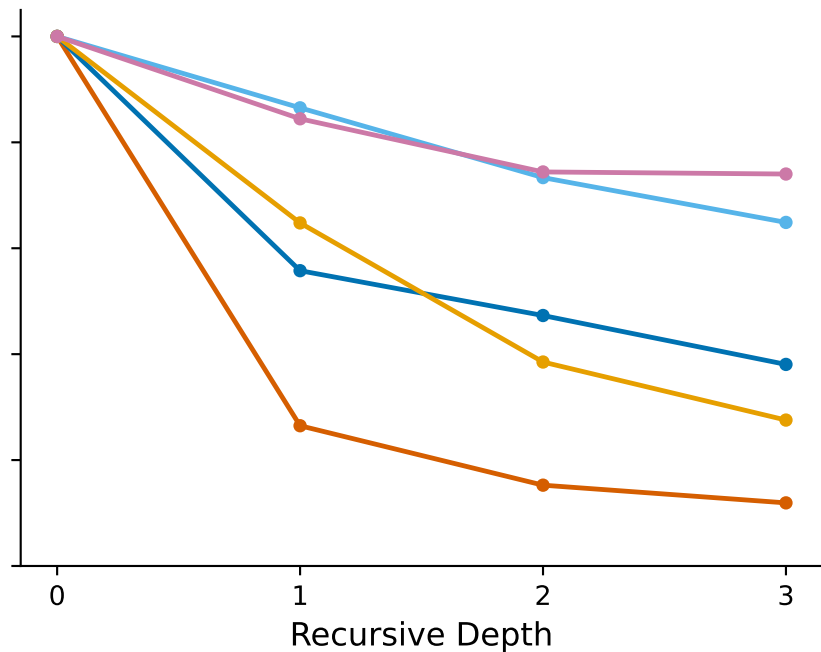
GPT-2 XL
