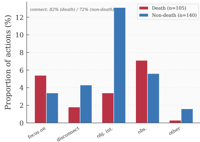
Internal (LLM)
