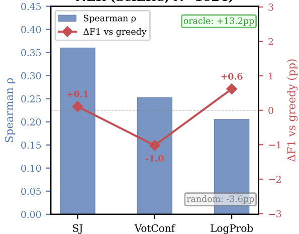
NER (SciERC, N=1024)
