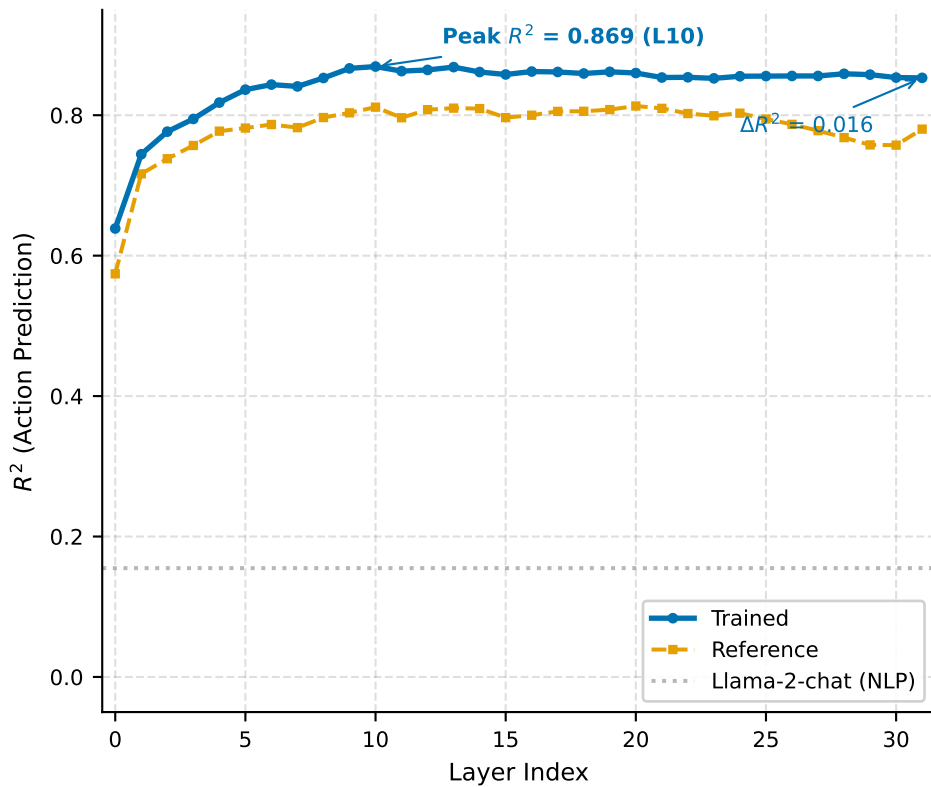
OpenVLA (VLA→VLA)
