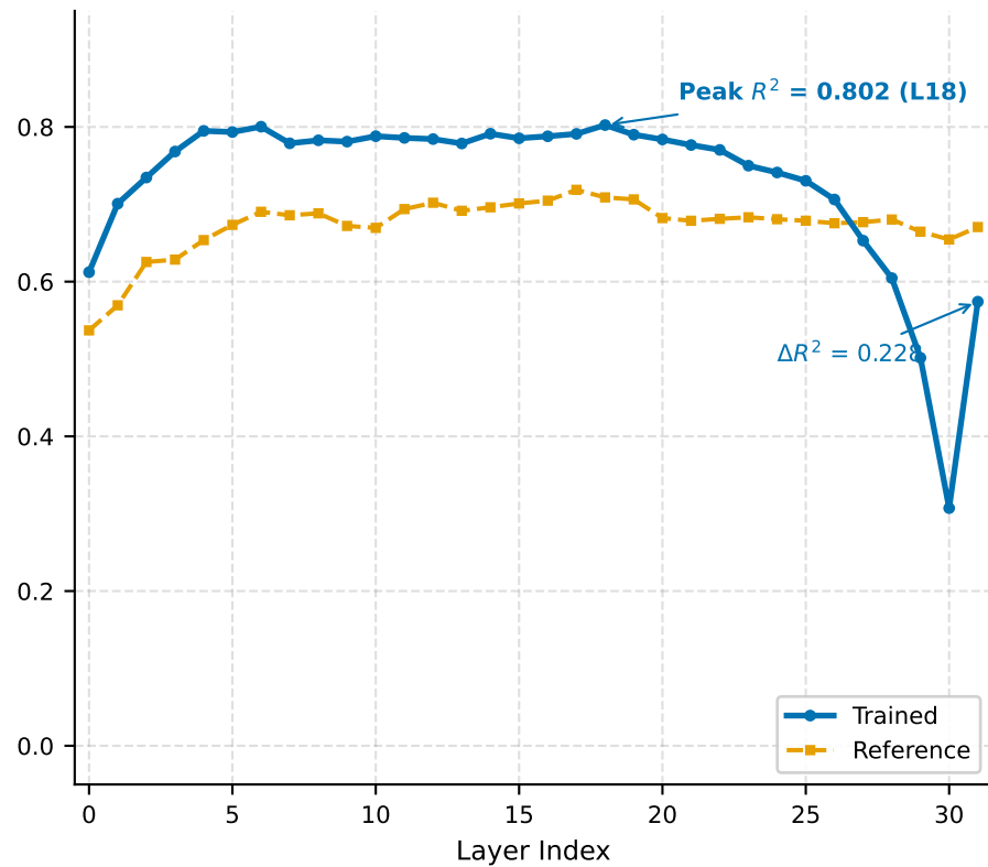
TracVLA (VLM→VLA)
