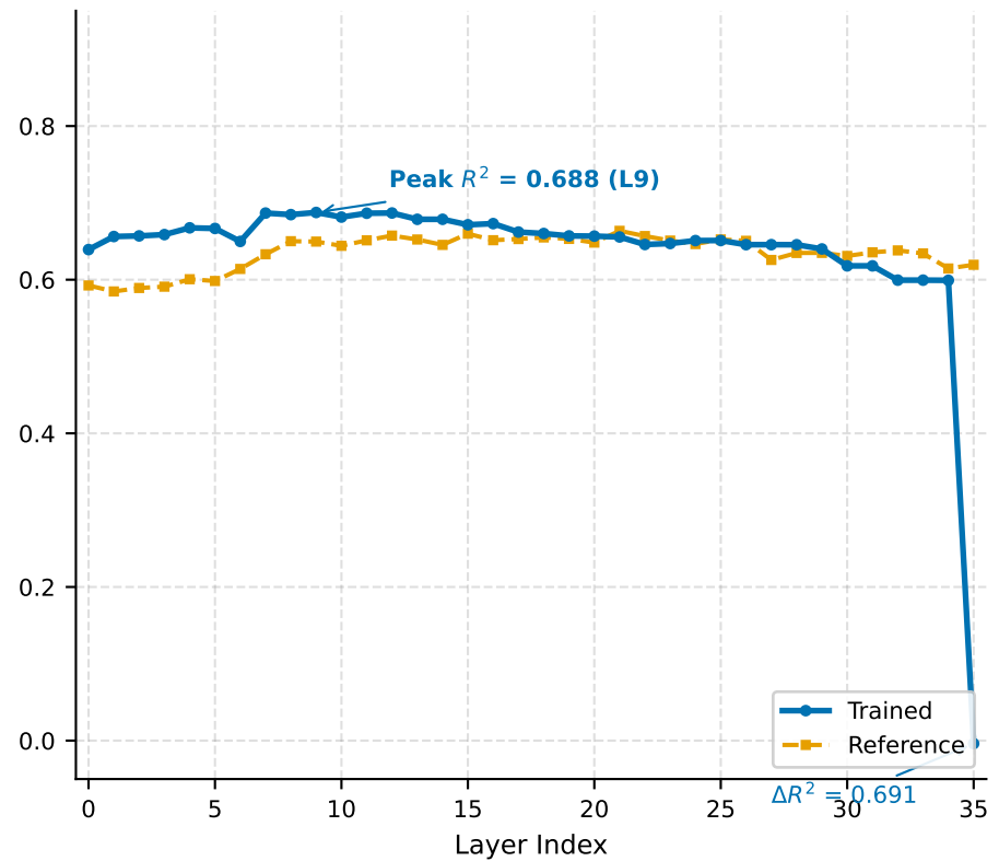
NORA (VLM→VLA)
